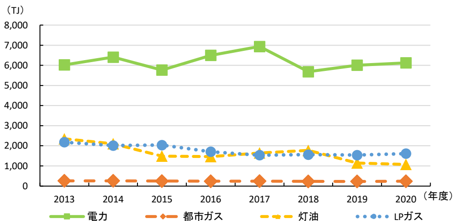
■家庭部門 燃料別エネルギー消費量の推移
