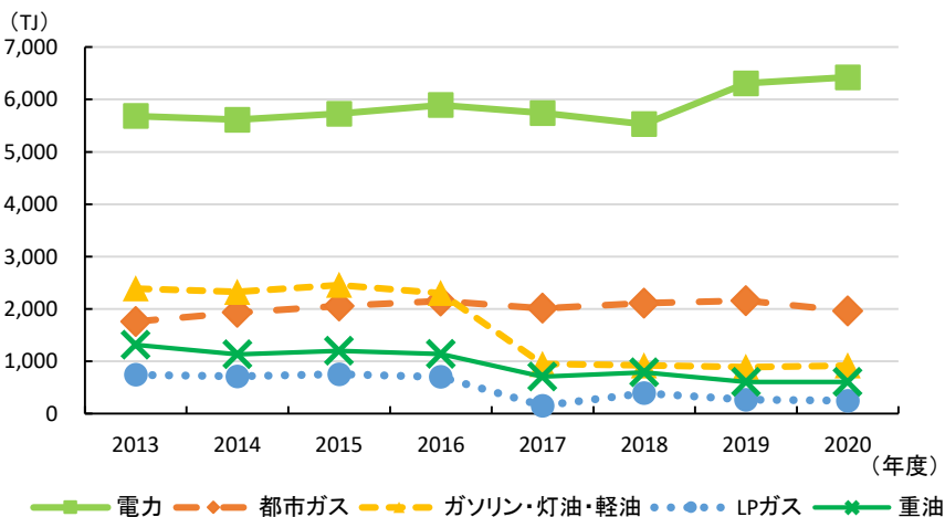
■業務部門 主要燃料別エネルギー消費量の推移
