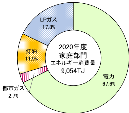
■家庭部門 燃料別エネルギー消費量
