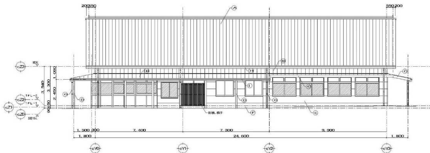
東立面图 1:100
