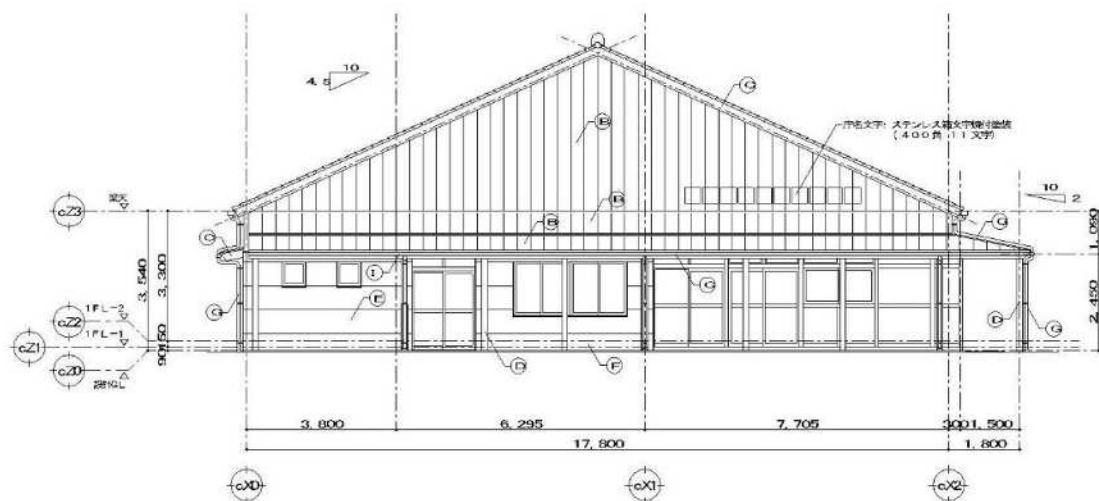
南立面图 1:100
