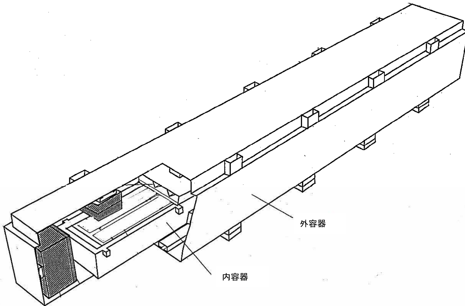
輸送容器概観図(NT-XII型)
