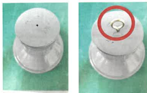
図7 強制通風筒KM-01の組み立て方(2/4)
