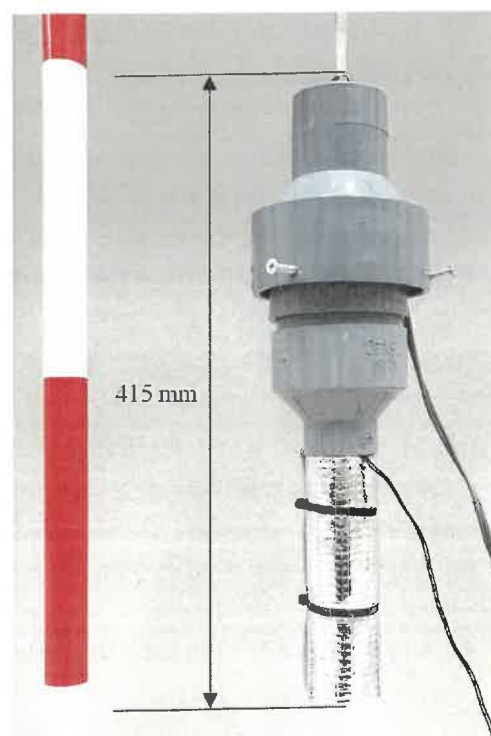
図1 強制通風筒 KM-01
