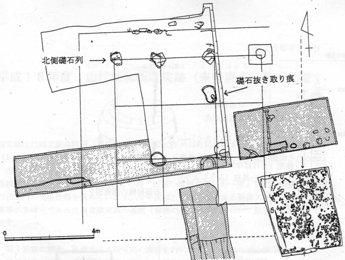
第1基壇トレンチ配置図 (S=1:100)
