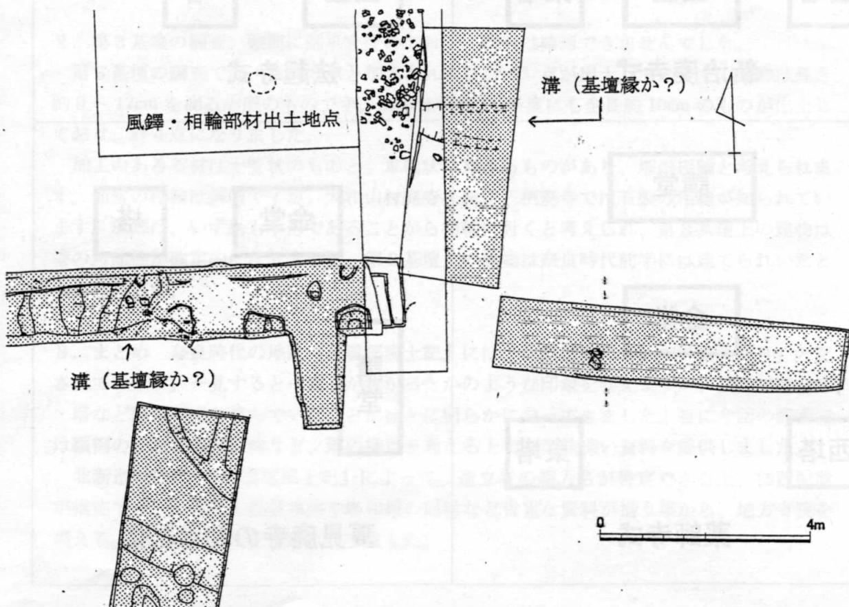
第3基壇トレンチ配置図 (S=1:100)
