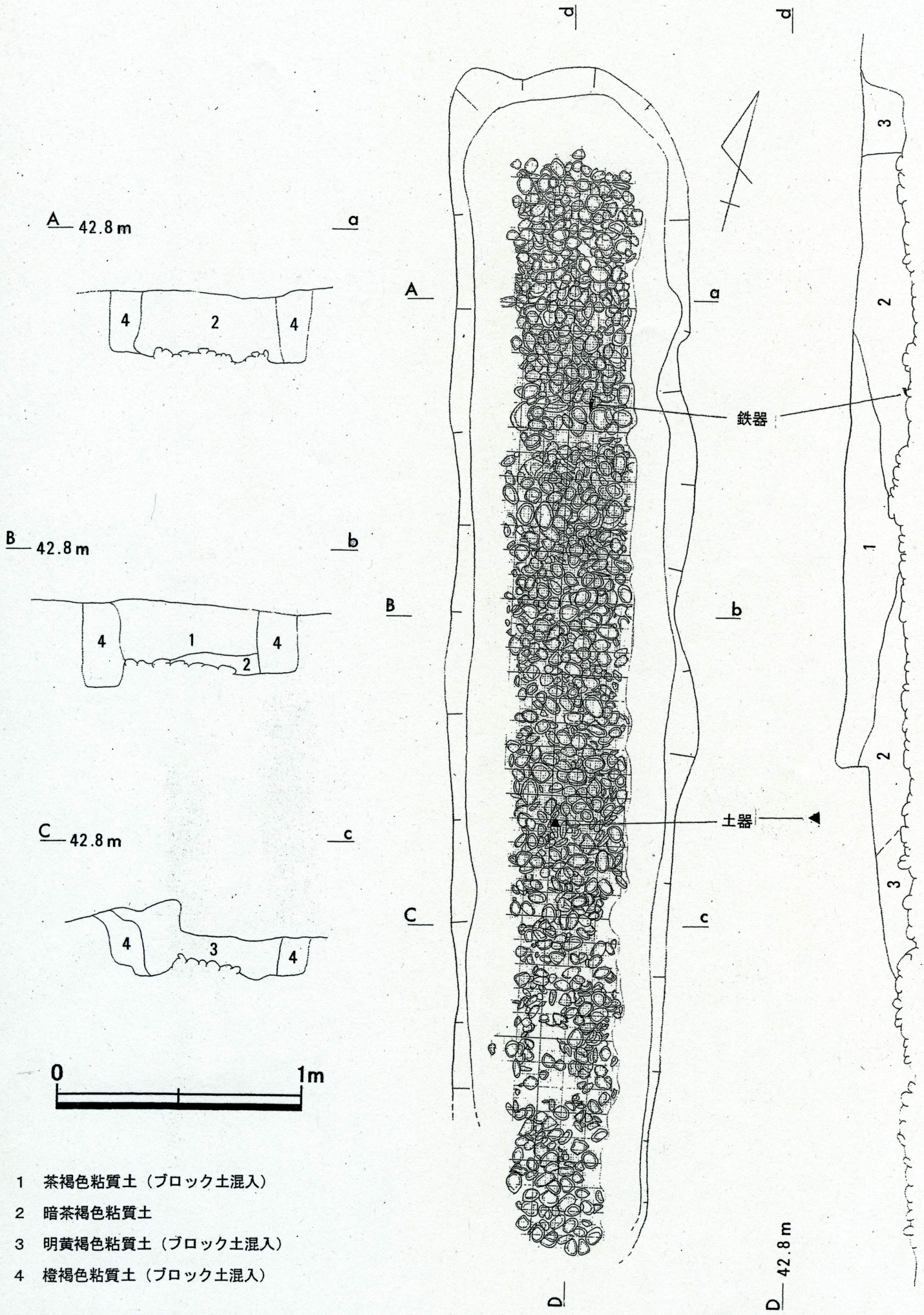
間谷東古墳主体部実測図 (S=1/20)
