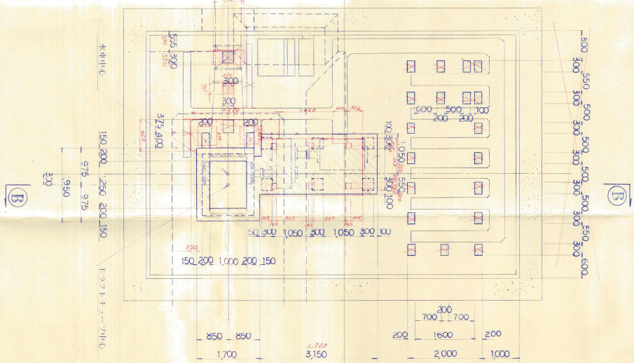
平面図
