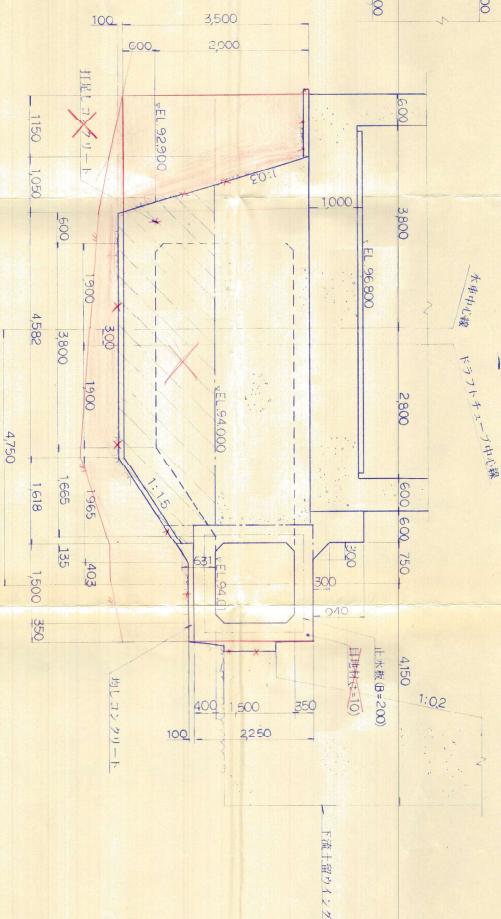
③-③ 断面図
