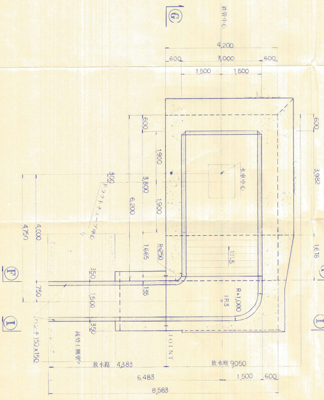
⑤-⑤ 断面図
