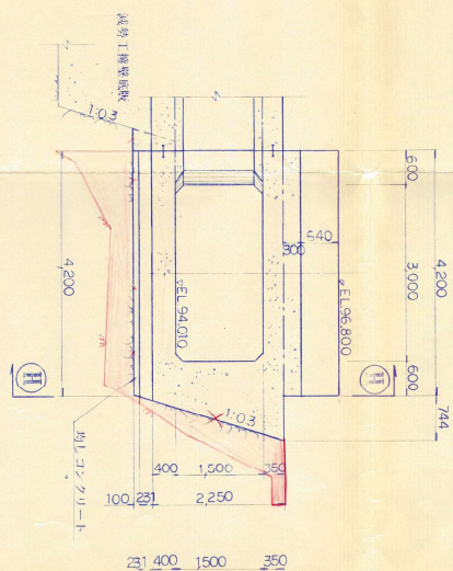
④-④ 断面図
