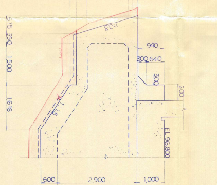
②-② 断面図
