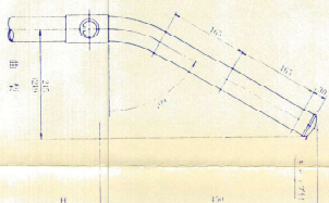
⑫ 網張りアイバー E=1/3
