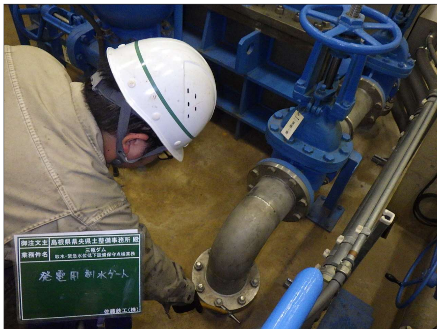
写真区分: 施工状況写真 工種: 発電用制水バルブ 種別: 充水装置 写真タイトル: ボルト緩み点 検状況 撮影箇所: 充水管
