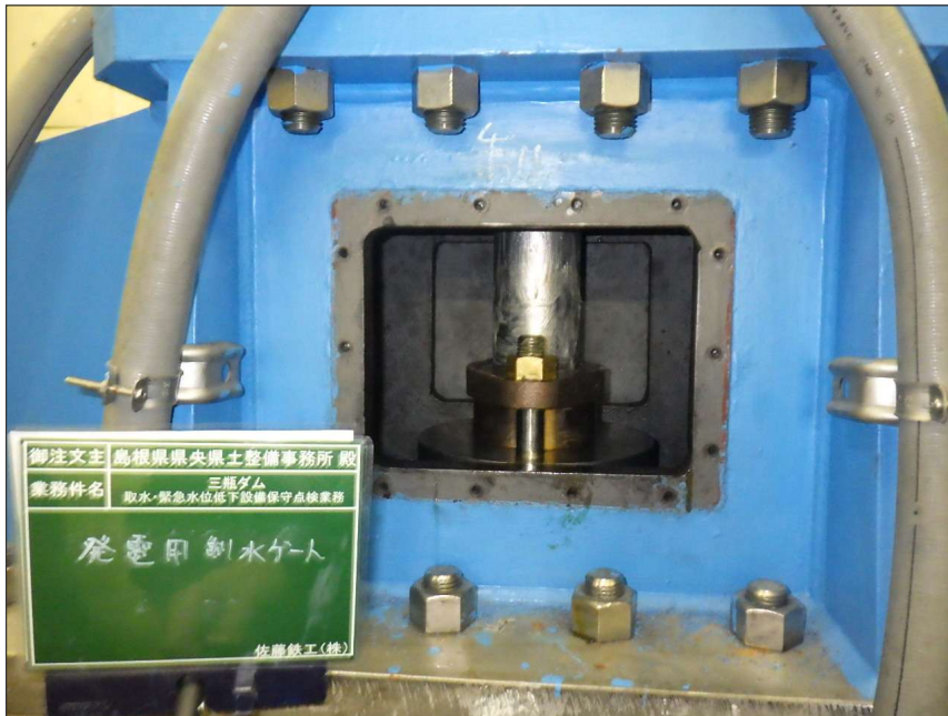
写真区分: 施工状況写真 工種: 発電用制水バルブ 種別: 開閉装置 写真タイトル: 給脂完了 撮影箇所: シリンダーロッド
