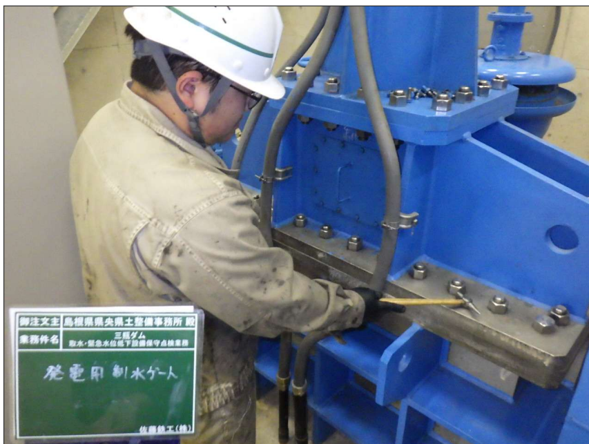
写真区分: 施工状況写真 工種: 発電用制水バルブ 種別: 開閉装置 写真タイトル: ボルト緩み点 検状況 撮影箇所: ボンネット
