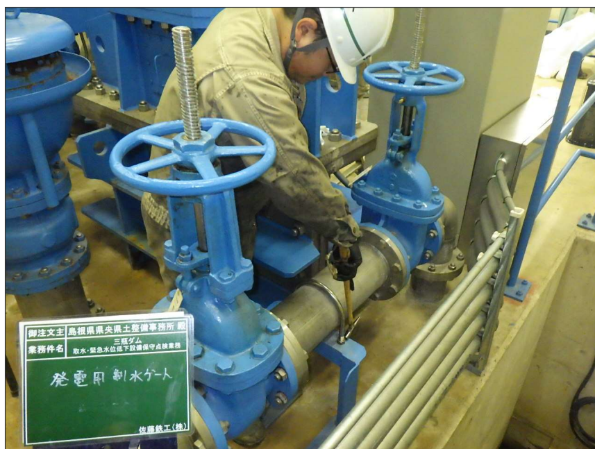
写真区分: 施工状況写真 工種: 発電用制水バルブ 種別: 充水装置 写真タイトル: ボルト緩み点 検状況 撮影箇所: 充水管架台
