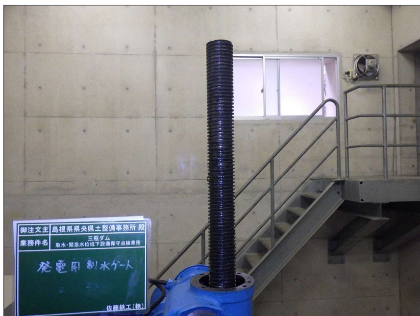
写真区分: 施工状況写真 工種: 発電用制水バルブ 種別: 開閉装置 写真タイトル: 給脂完了 撮影箇所: スピンドル
