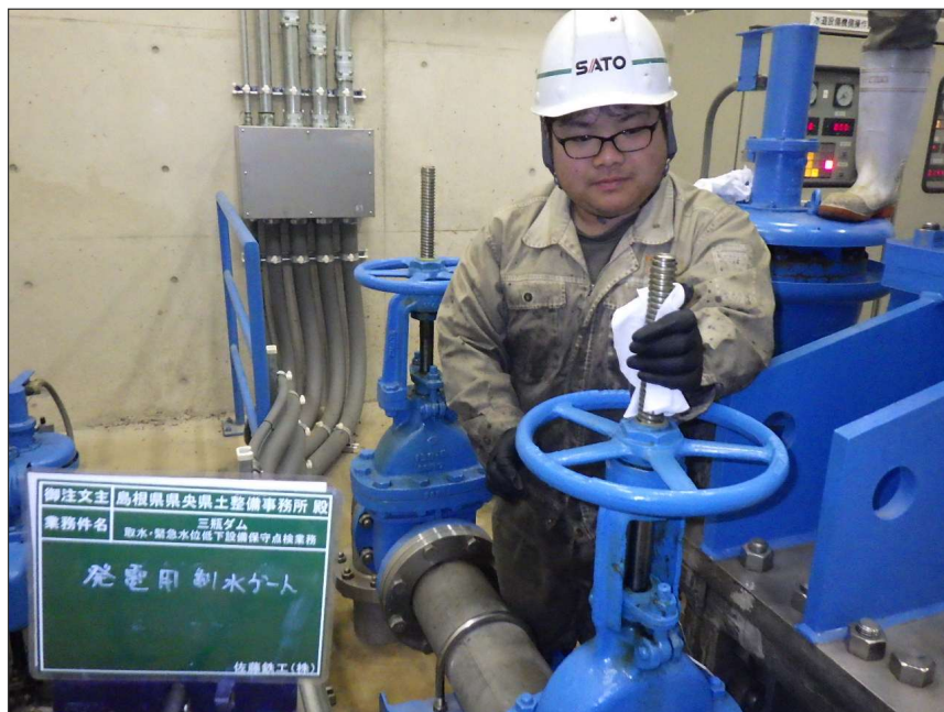
写真区分: 施工状況写真 工種: 発電用制水バルブ 種別: 充水装置 写真タイトル: 清掃状況 撮影箇所: スピンドル
