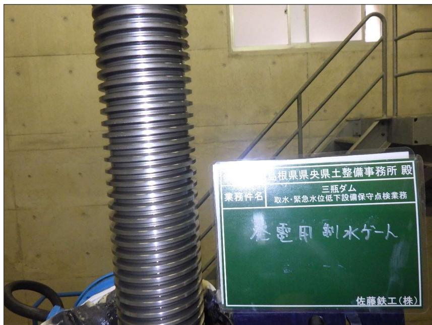
写真区分: 施工状況写真 工種: 発電用制水バルブ 種別: 開閉装置 写真タイトル: 歯面確認 撮影箇所: スピンドル
