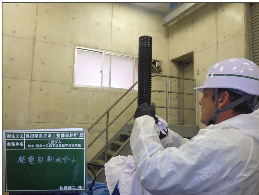
写真区分: 施工状況写真 工種: 発電用制水バルブ 種別: 開閉装置 写真タイトル: 清掃状況 撮影箇所: スピンドル
