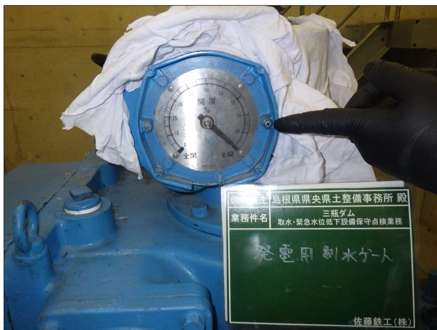
写真区分: 施工状況写真 工種: 発電用制水バルブ 種別: 開閉装置 写真タイトル: 全閉確認 撮影箇所: 開度計
