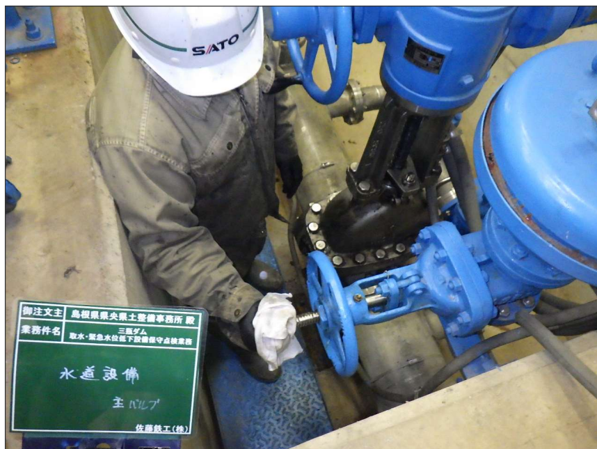
写真区分: 施工状況写真 工種: 水道設備 種別: 主バルブ 細別: 充水装置 写真タイトル: 清掃状況 撮影箇所: スピンドル
