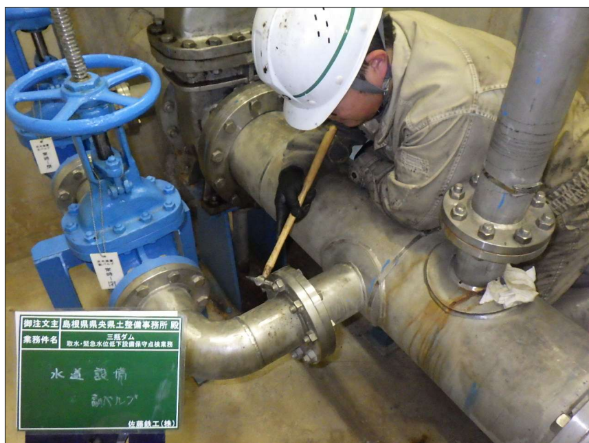
写真区分: 施工状況写真 工種: 水道設備 種別: 副バルブ 写真タイトル: ボルト緩み点 検状況 撮影箇所: 充水管
