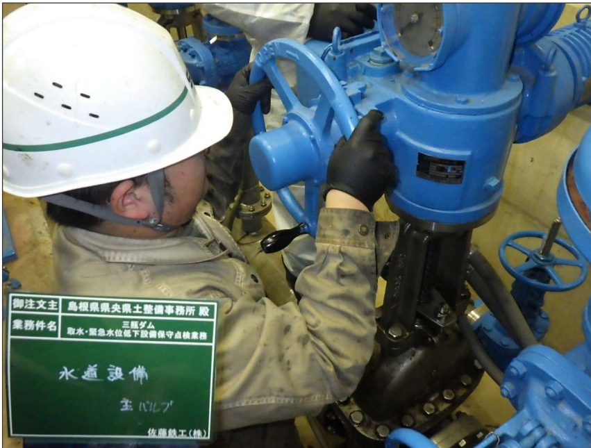
写真区分: 施工状況写真 工種: 水道設備 種別: 主バルブ 写真タイトル: 機能確認 撮影箇所: 手動ハンドル
