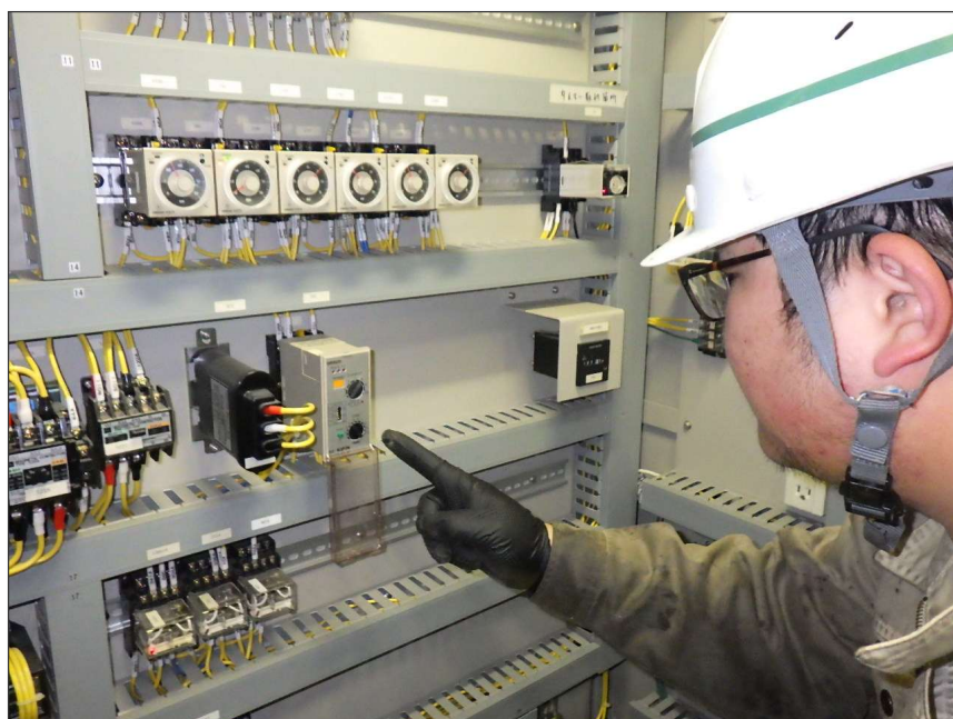
写真区分: 施工状況写真 工種: 水道設備 種別: 機側操作盤 写真タイトル: 設定値確認状況 撮影箇所: 3Eリレー
