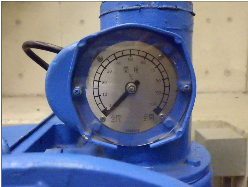
写真区分: 施工状況写真 工種: 水道設備 種別: 主バルブ 写真タイトル: 全閉確認
