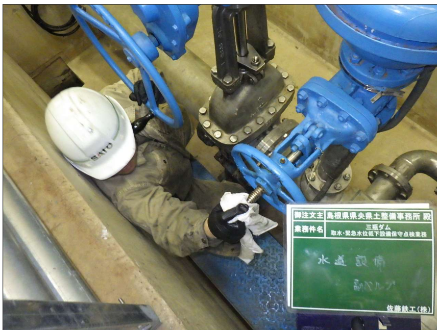
写真区分: 施工状況写真 工種: 水道設備 種別: 副バルブ 細別: 充水装置 写真タイトル: 清掃状況 撮影箇所: スピンドル
