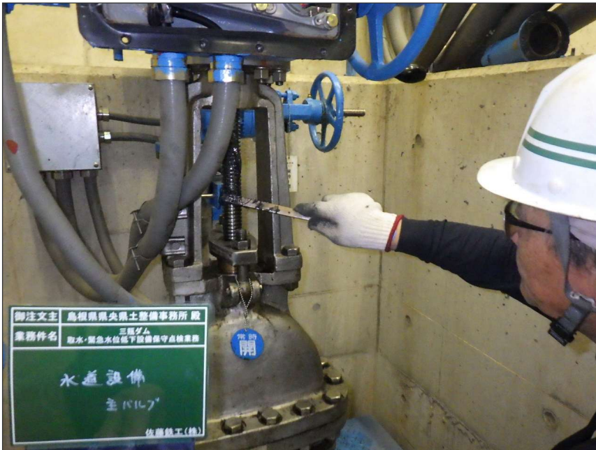
写真区分: 施工状況写真 工種: 水道設備 種別: 主バルブ 写真タイトル: 給脂状況 撮影箇所: スピンドル
