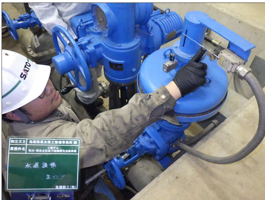
写真区分: 施工状況写真 工種: 水道設備 種別: 主バルブ 細別: 充水装置 写真タイトル: 外観点検状況 撮影箇所: 充水管
