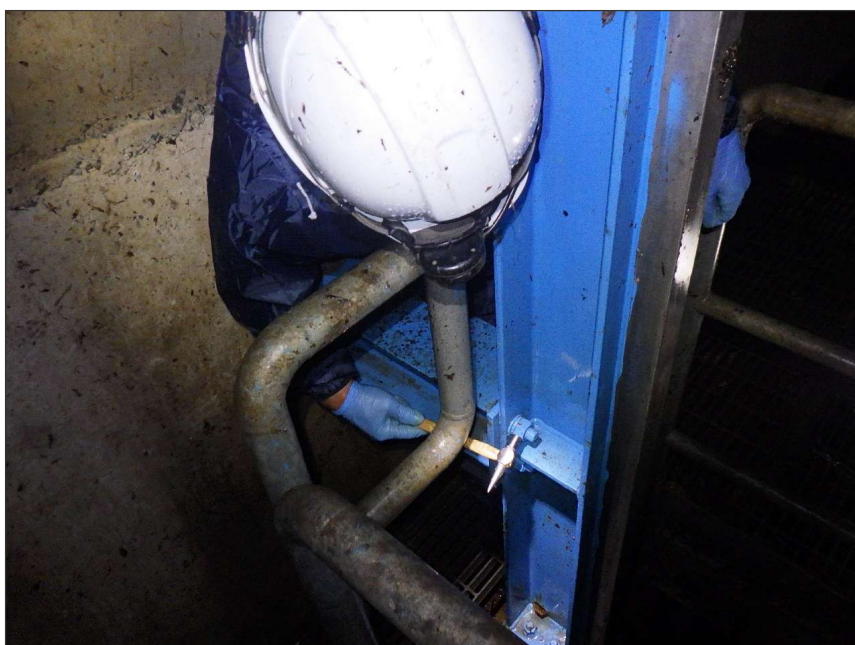
写真区分: 施工状況写真 工種: 制水ゲート 種別: 扉体 細別: 戸当り 写真タイトル: ボルト緩み点 検状況 撮影箇所: 戸当り
