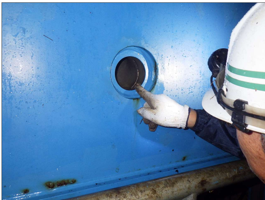
写真区分: 施工状況写真 工種: 制水ゲート 種別: 扉体 写真タイトル: 外観点検状況 撮影箇所: 充水管
