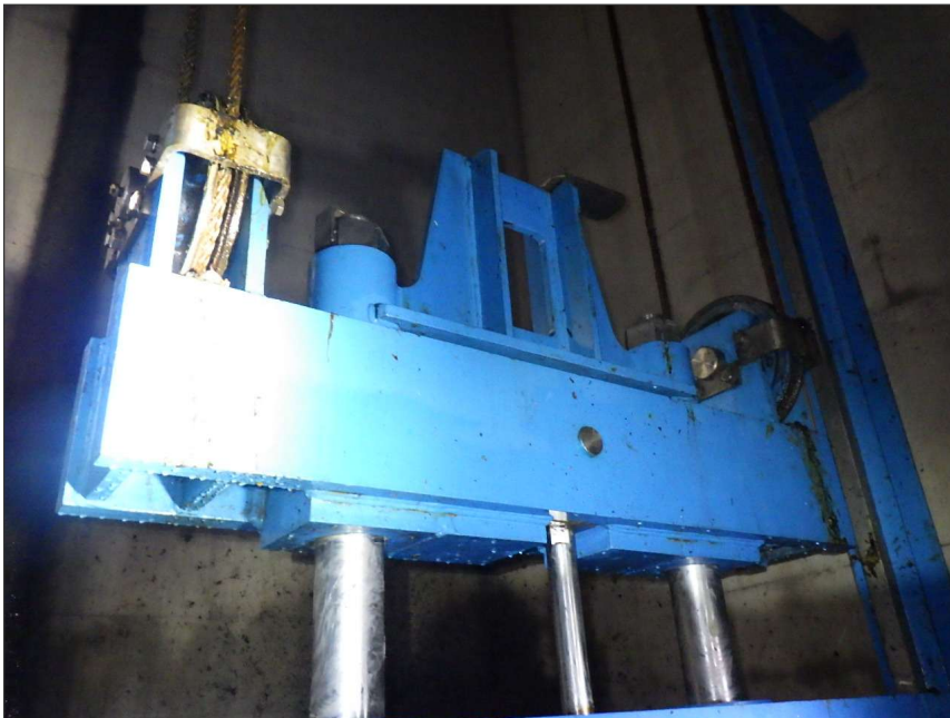
写真区分: 施工状況写真 工種: 制水ゲート 種別: 扉体 細別: リフティングビーム 写真タイトル: 外観点検状況 撮影箇所: リフティングビーム
