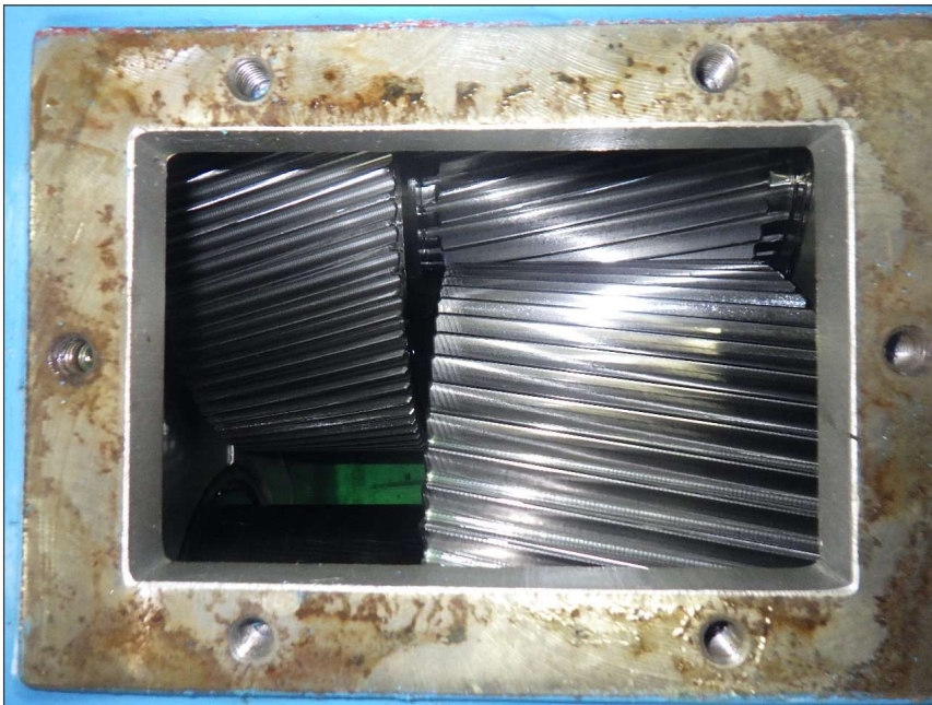
写真区分: 施工状況写真 工種: 制水ゲート 種別: 開閉装置 細別: 減速機 写真タイトル: 歯面確認 撮影箇所: 減速機
