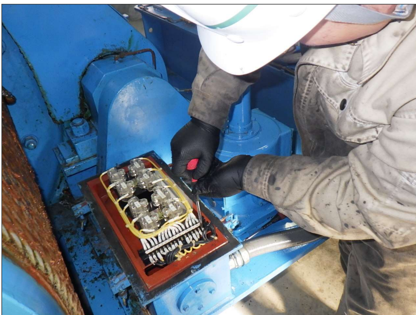
写真区分: 施工状況写真 工種: 制水ゲート 種別: 開閉装置 細別: 開度計・制限開閉器 写真タイトル: 端子緩み点検 状況 撮影箇所: 制限開閉器
