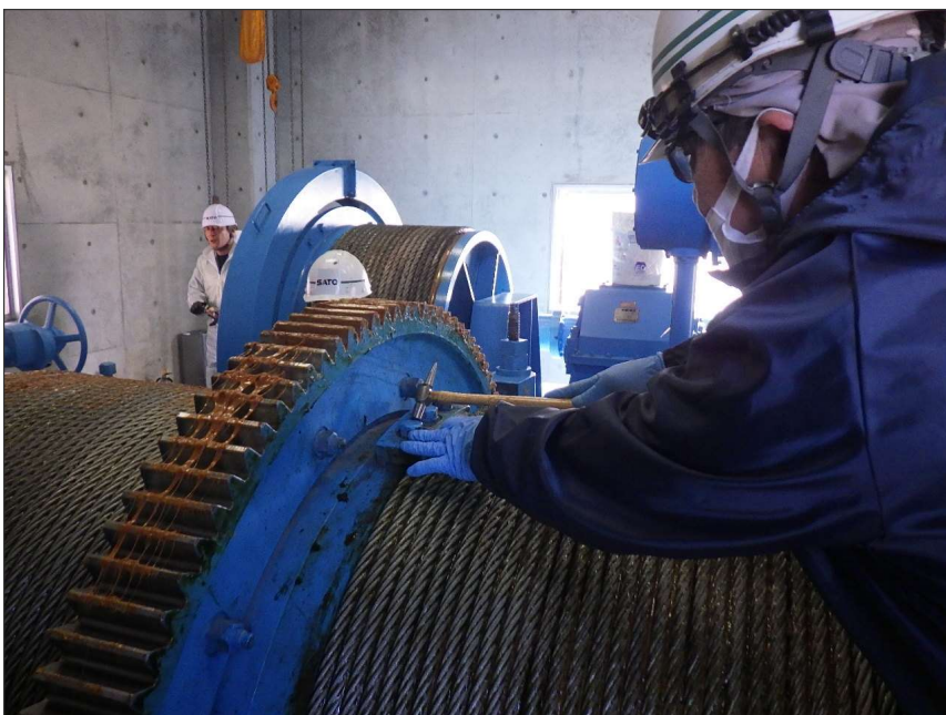
写真区分: 施工状況写真 工種: 制水ゲート 種別: 開閉装置 写真タイトル: ボルト緩み点 検状況 撮影箇所: ロープ端末締付ボルト
