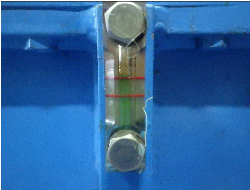
写真区分: 施工状況写真 工種: 制水ゲート 種別: 開閉装置 細別: 減速機 写真タイトル: 抜油前 撮影箇所: 油面計
