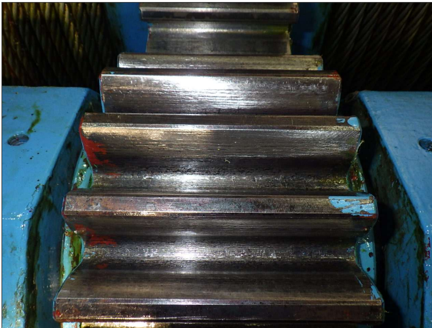
写真区分: 施工状況写真 工種: 制水ゲート 種別: 開閉装置 写真タイトル: 歯面確認 撮影箇所: ドラムギヤ
