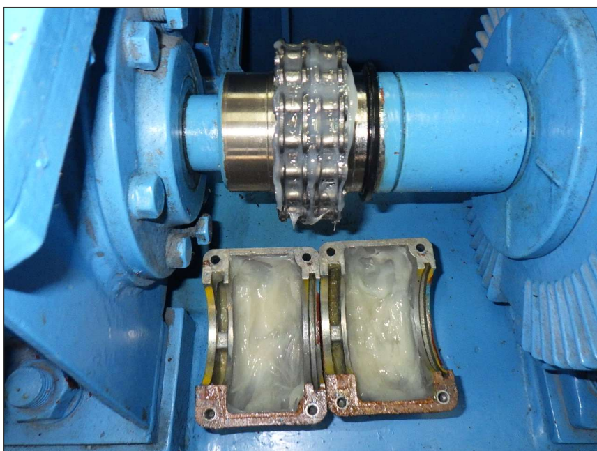
写真区分: 施工状況写真 工種: 制水ゲート 種別: 開閉装置 写真タイトル: 給脂完了 撮影箇所: チェーンカップリング
