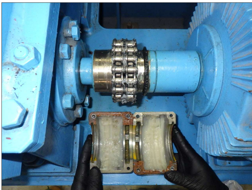
写真区分: 施工状況写真 工種: 制水ゲート 種別: 開閉装置 写真タイトル: 清掃前 撮影箇所: チェーンカップリング
