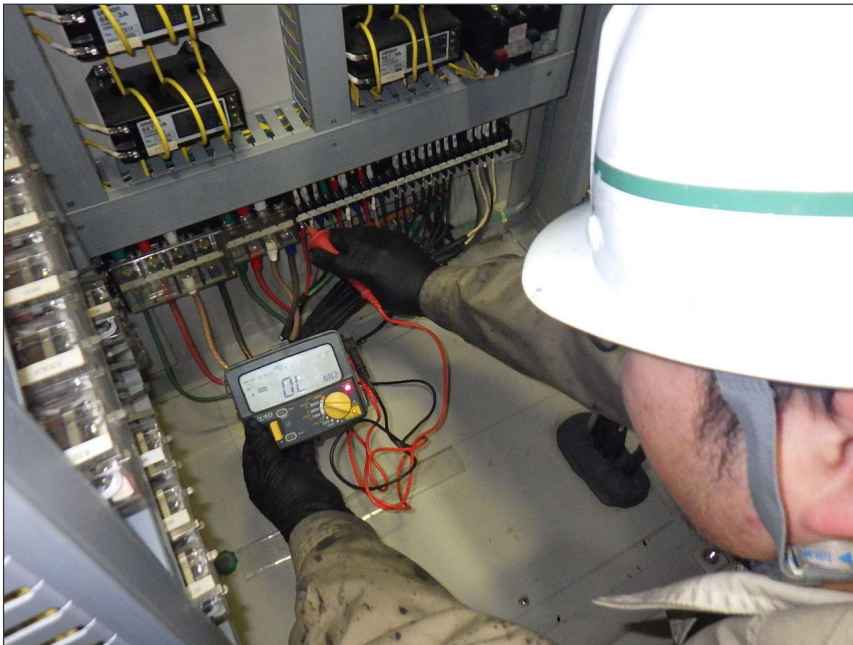
写真区分: 施工状況写真 工種: 制水ゲート 種別: 開閉装置 写真タイトル: 絶縁抵抗測定 状況 撮影箇所: 機側操作盤
