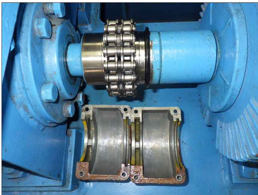
写真区分: 施工状況写真 工種: 制水ゲート 種別: 開閉装置 写真タイトル: 清掃完了 撮影箇所: チェーンカップリング
