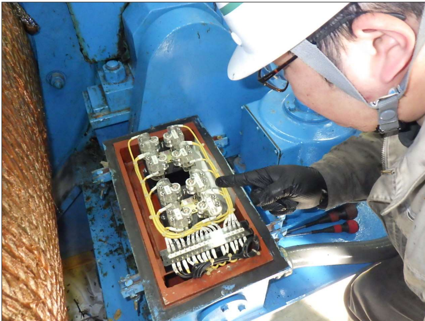
写真区分: 施工状況写真 工種: 制水ゲート 種別: 開閉装置 細別: 開度計・制限開閉器 写真タイトル: 外観点検状況 撮影箇所: 制限開閉器
