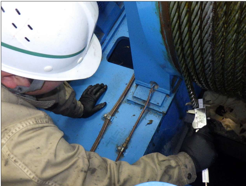
写真区分: 施工状況写真 工種: 制水ゲート 種別: 開閉装置 写真タイトル: 計測状況 撮影箇所: ワイヤロープ径
