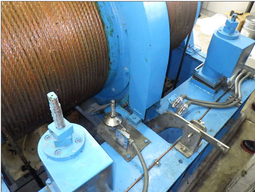
写真区分: 施工状況写真 工種: 制水ゲート 種別: 開閉装置 細別: ゲートロボ 写真タイトル: 給脂完了 撮影箇所: スピンドル
