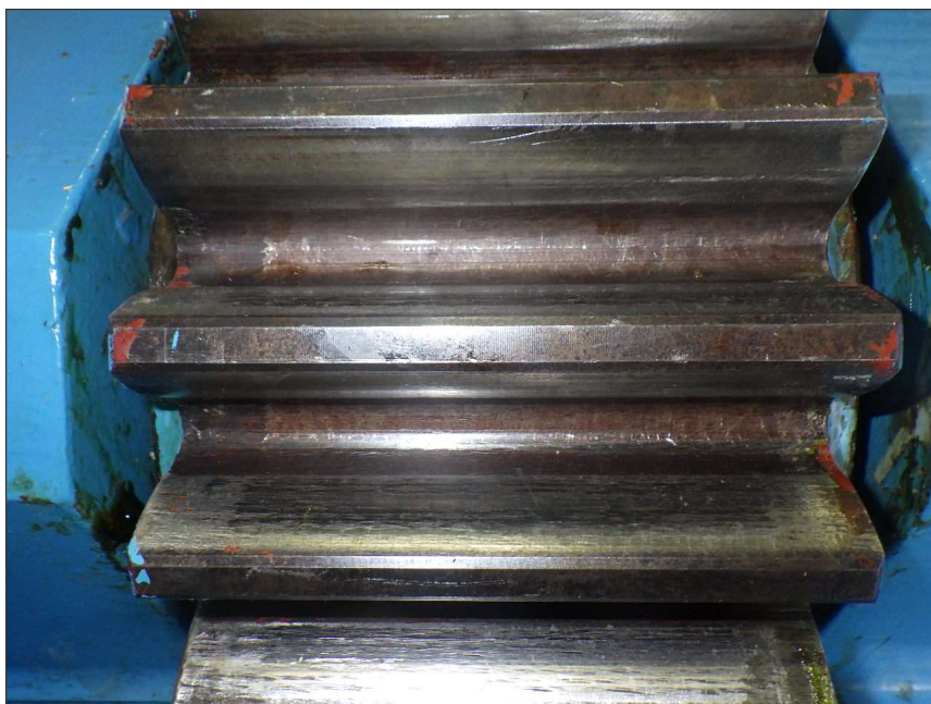
写真区分: 施工状況写真 工種: 取水ゲート 種別: 開閉装置 写真タイトル: 歯面確認 撮影箇所: ドラムギヤ
