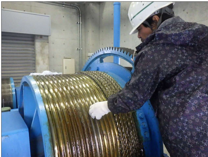
写真区分: 施工状況写真 工種: 取水ゲート 種別: 開閉装置 写真タイトル: 清掃状況 撮影箇所: ワイヤドラム
