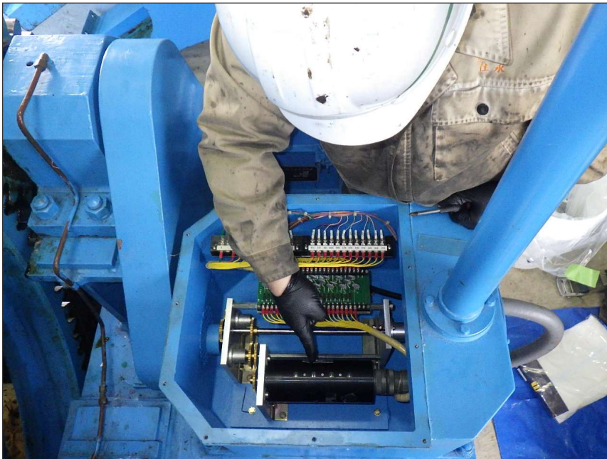
写真区分: 施工状況写真 工種: 取水ゲート 種別: 開閉装置 細別: 制限開閉器 写真タイトル: 外観点検状況 撮影箇所: 制限開閉器
