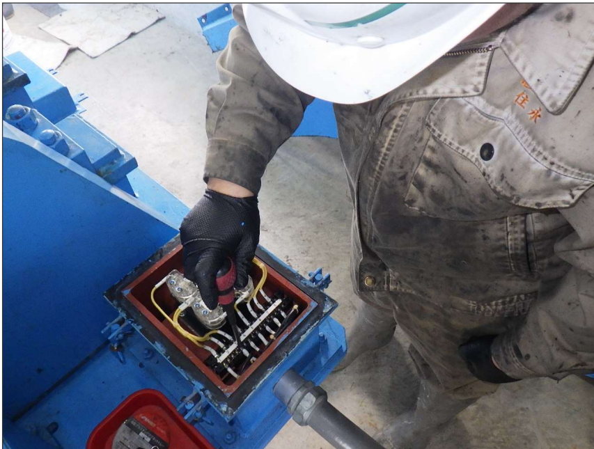
写真区分: 施工状況写真 工種: 取水ゲート 種別: 開閉装置 細別: 制限開閉器 写真タイトル: 端子緩み点検 状況 撮影箇所: 制限開閉器
