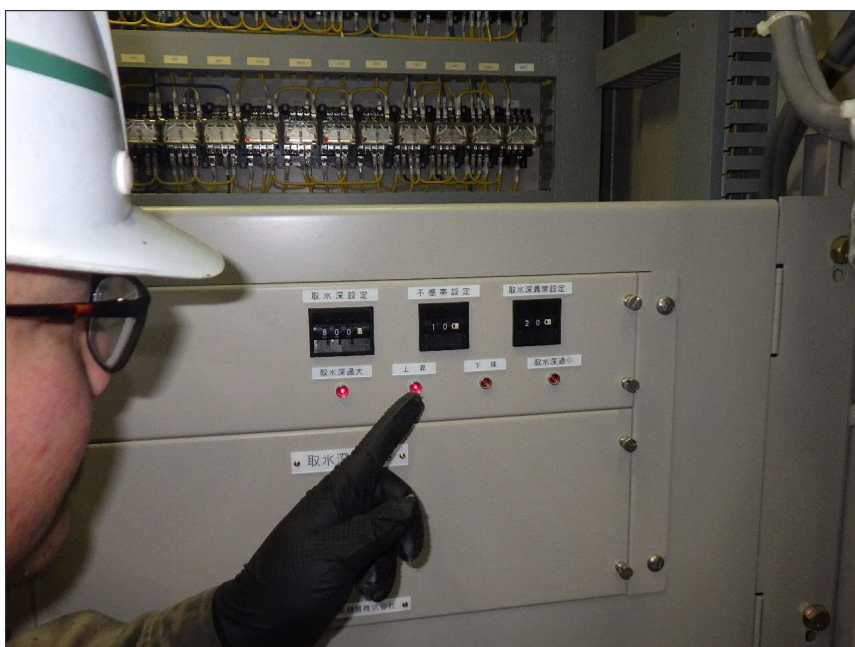
写真区分: 施工状況写真 工種: 取水ゲート 種別: 開閉装置 写真タイトル: 設定値確認状 況 撮影箇所: 機側操作盤
