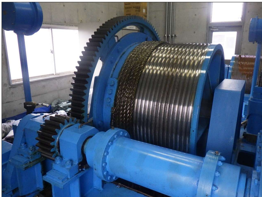
写真区分: 施工状況写真 工種: 取水ゲート 種別: 開閉装置 写真タイトル: 清掃完了 撮影箇所: ワイヤドラム・ドラムギヤ
