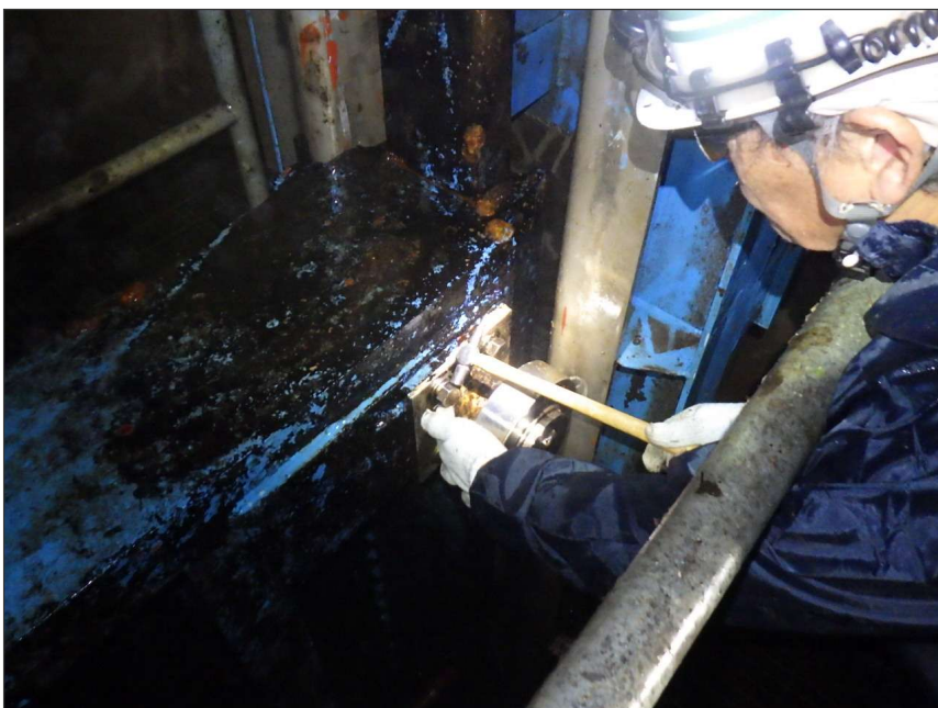
写真区分: 施工状況写真 工種: 取水ゲート 種別: 扉体 写真タイトル: ボルト緩み点 検状況 撮影箇所: サイドローラ
