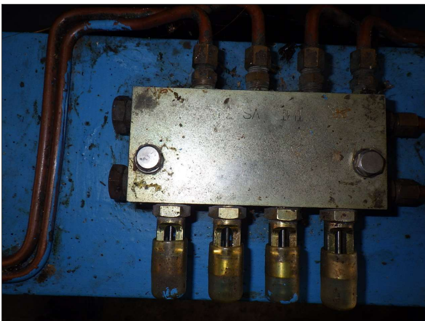
写真区分: 施工状況写真 工種: 取水ゲート 種別: 開閉装置 写真タイトル: 給脂完了 撮影箇所: 集中給油装置
