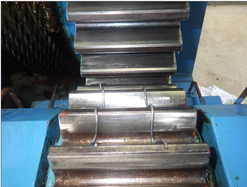
写真区分: 施工状況写真 工種: 取水ゲート 種別: 開閉装置 写真タイトル: 計測状況 撮影箇所: バックラッシ測定 検体
