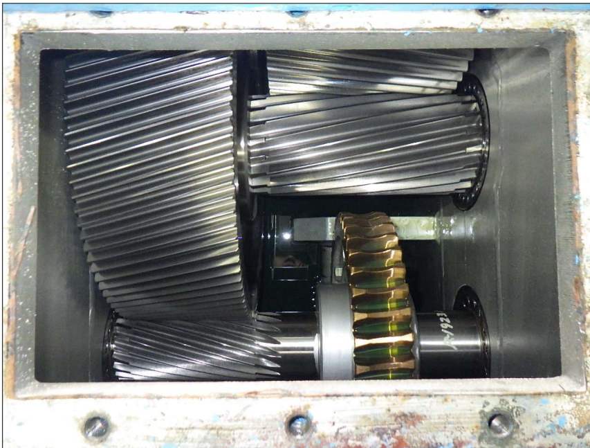
写真区分: 施工状況写真 工種: 取水ゲート 種別: 開閉装置 細別: 減速機 写真タイトル: 歯面確認 撮影箇所: 減速機
