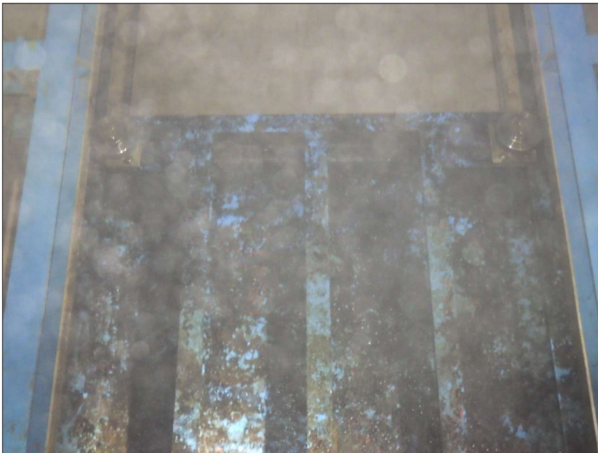
写真区分: 施工状況写真 工種: 取水ゲート 種別: 扉体 写真タイトル: 外観点検状況 撮影箇所: サイドローラ
