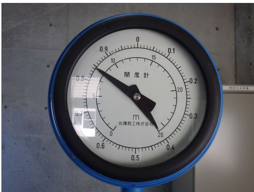
写真区分: 施工状況写真 工種: 取水ゲート 種別: 開閉装置 写真タイトル: 全開確認 撮影箇所: 開度計
