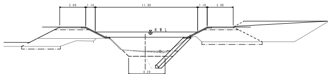
断面図 NO. 21付近
