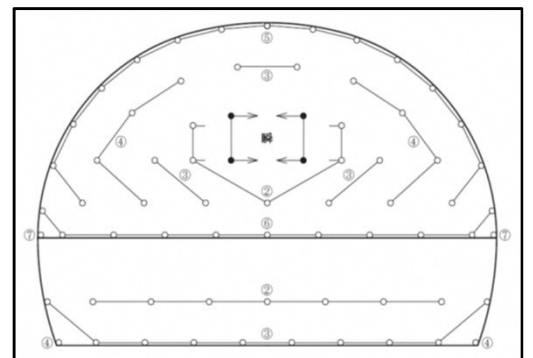
発破計画書
