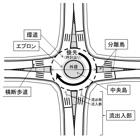
ラウンドアバウト標準図
