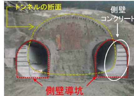
施工状況(側壁導坑完了)
