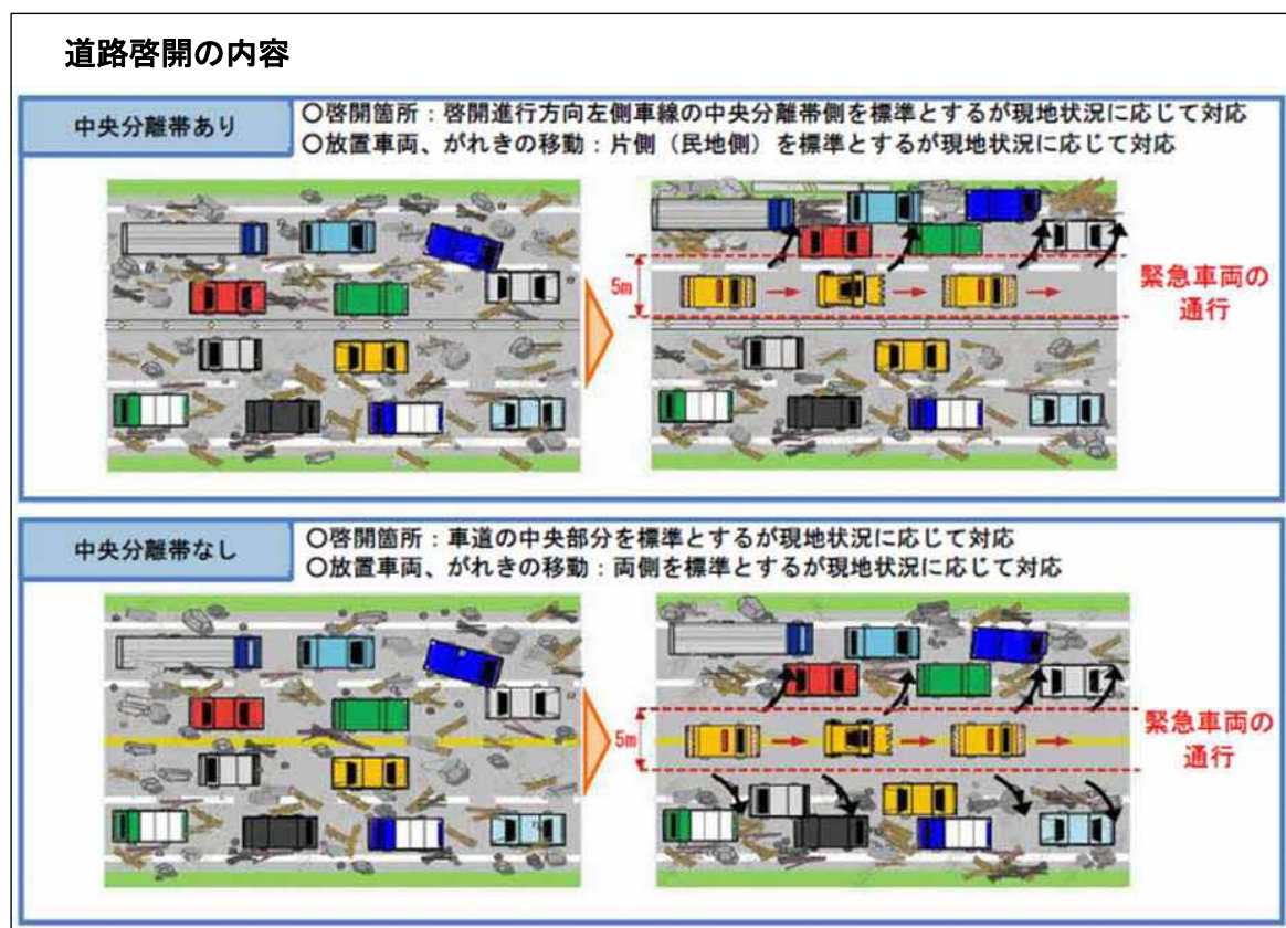
図IV-7 道路啓開の作業内容
