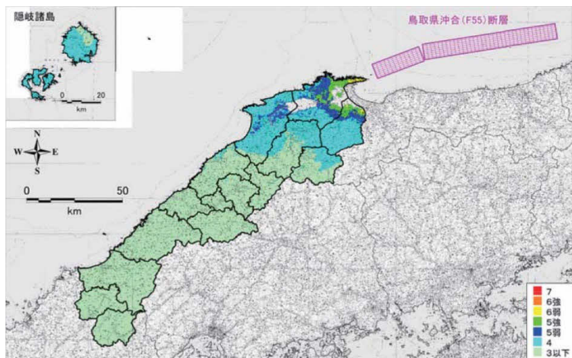
鳥取県沖合(F55)断層 (M8.1)
