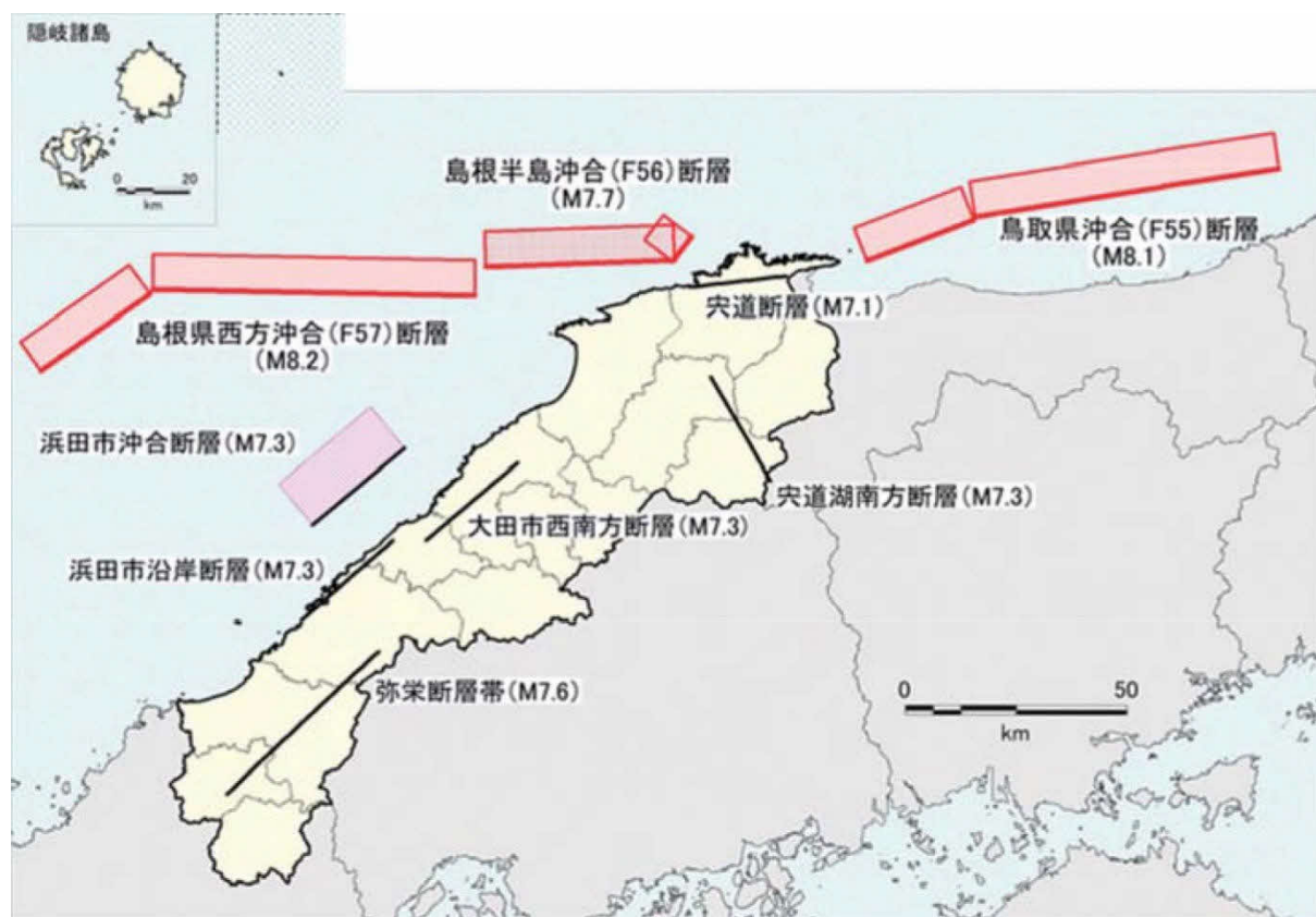
図Ⅱ-13 地震動の想定を対象とした地震の断層位置
