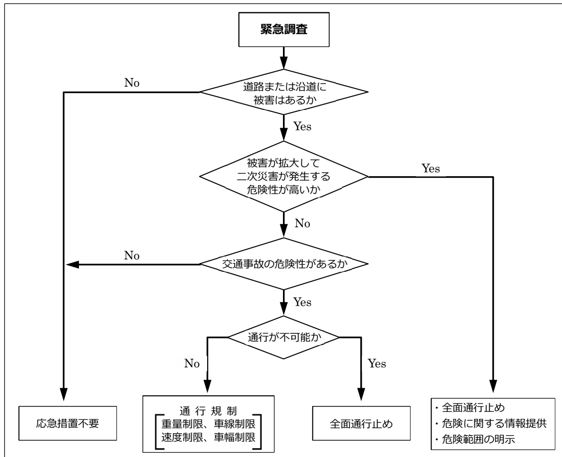
図IV-4 道路施設における緊急措置の流れ
