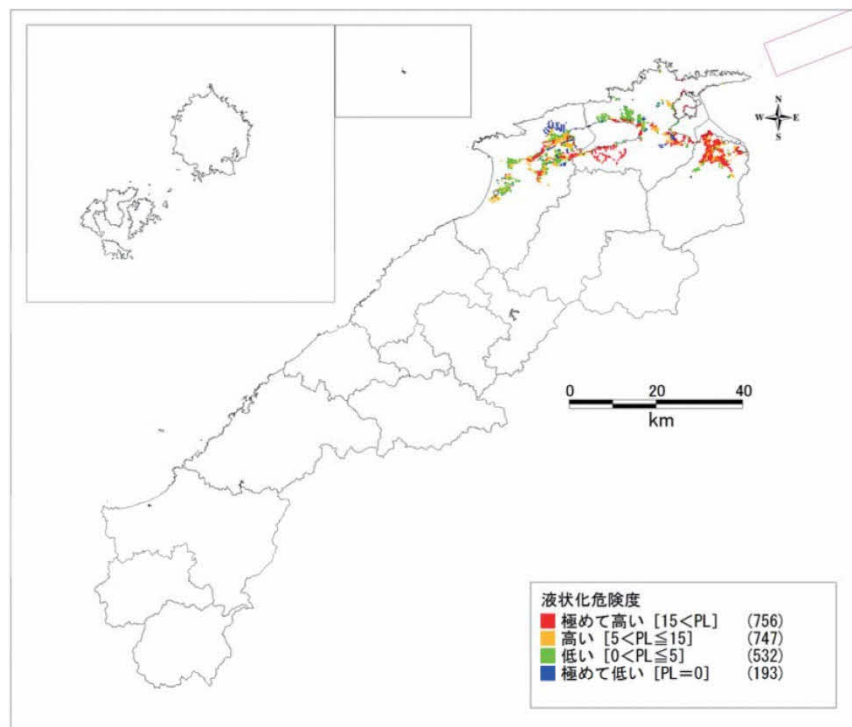
図Ⅱ-15 各地震における液状化危険度分布⑥
