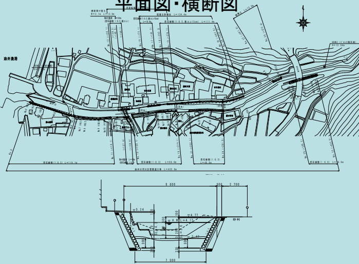
平面図・横断図
