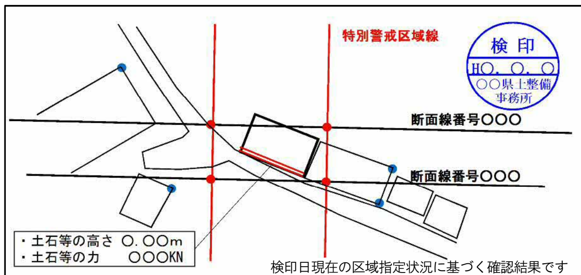
土石流の例
