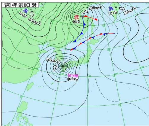
令和4年9月19日の天気図
