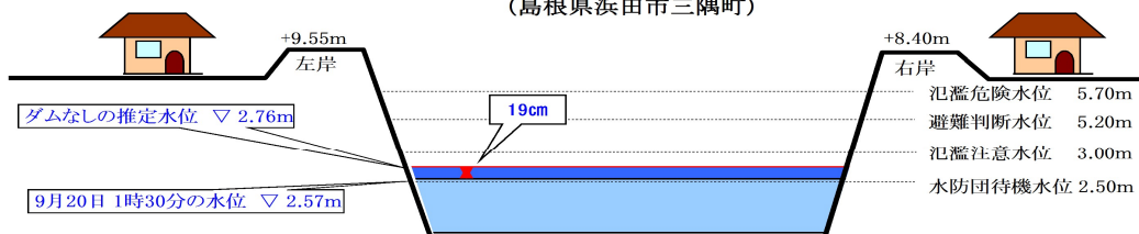
三隅水位局付近断面図 (島根県浜田市三隅町)
