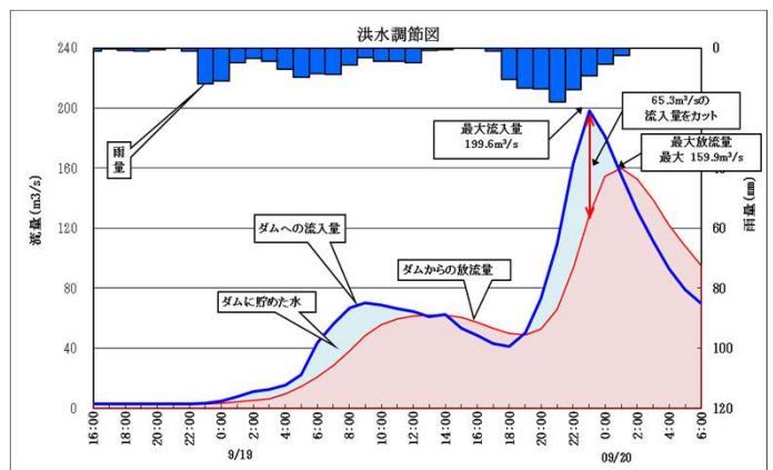
9月19日～20日の洪水調節図
