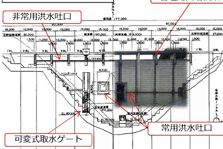
御部ダムを川の下流から見た図
