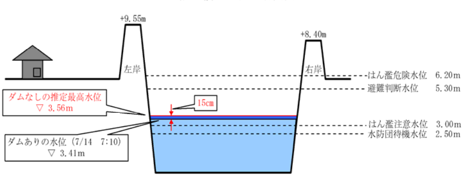
洪水調節図
