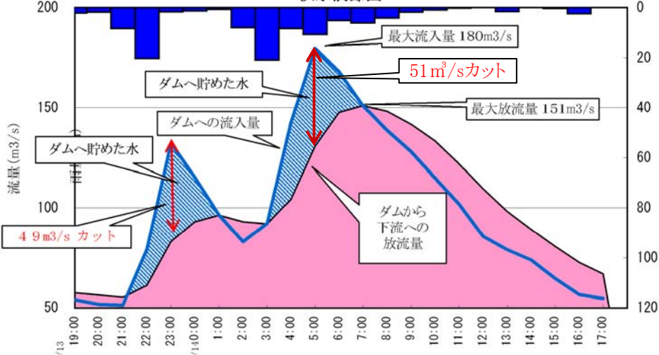
洪水調節図
