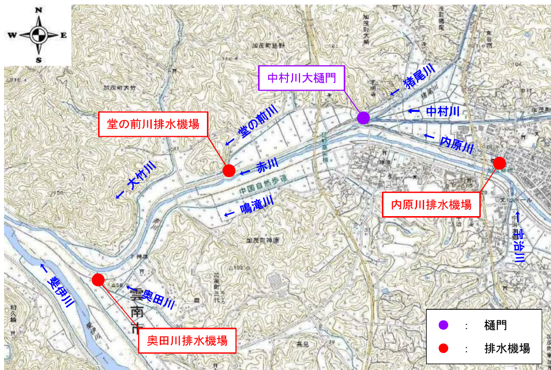
図-4.3 本整備計画の対象河川管理施設の位置図
