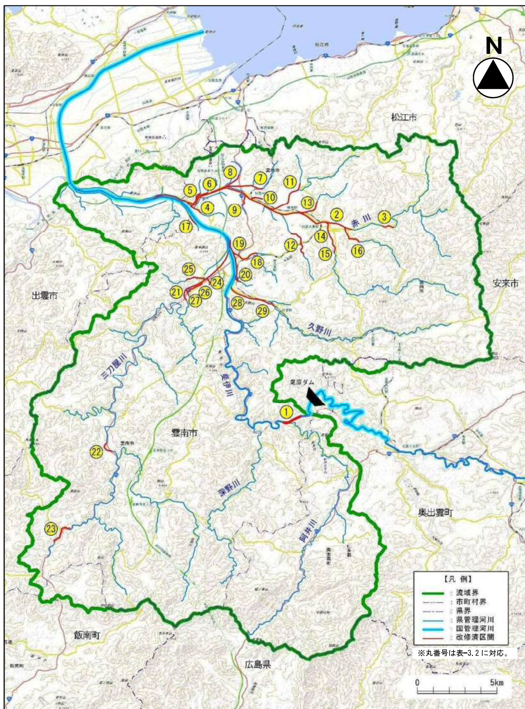
図-3.1 河川改修整備状況
