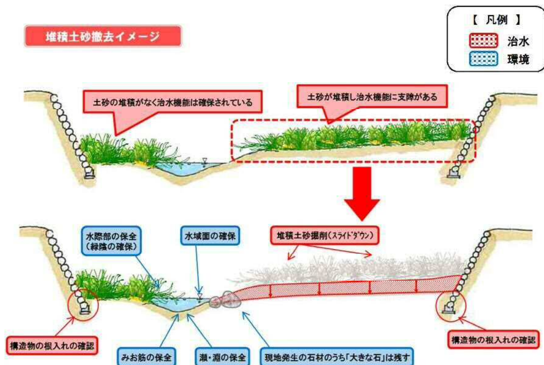
図-4.4 堆積土砂撤去イメージ図
