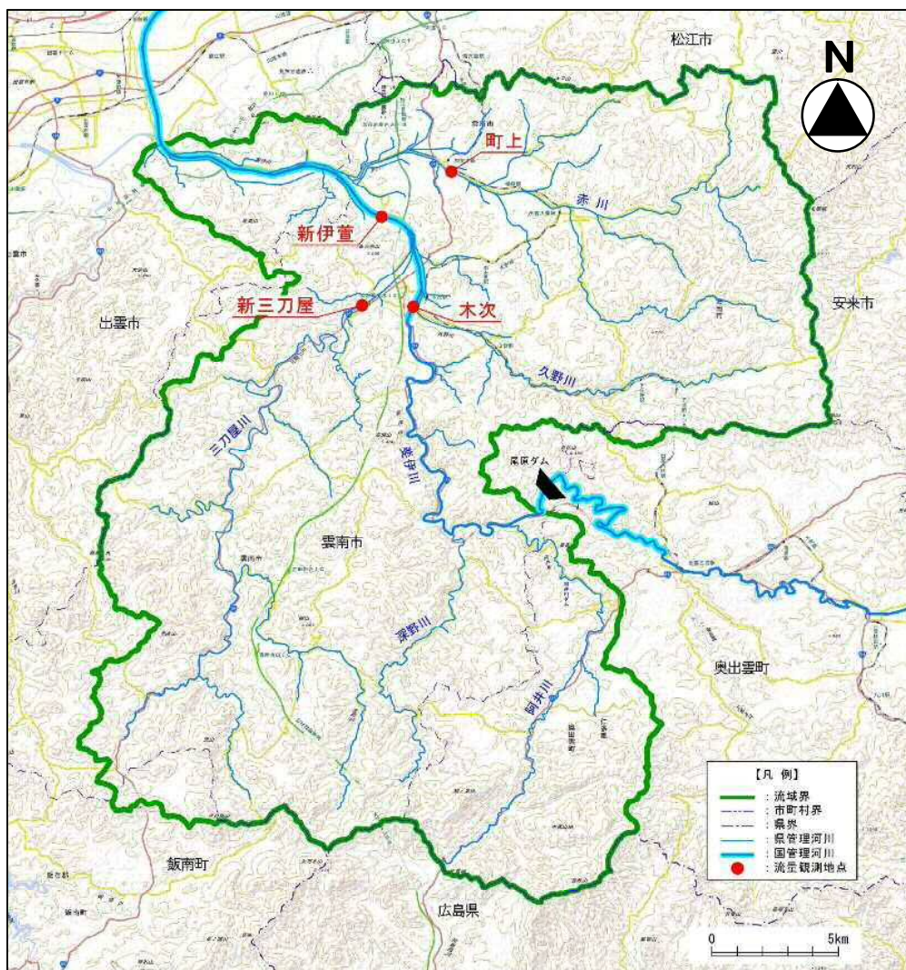
図-3.3 流量観測地点位置図
