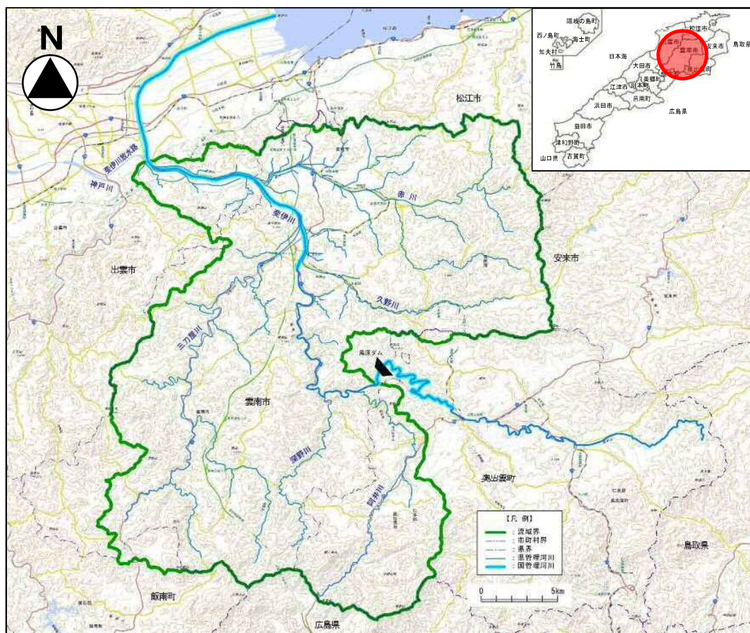
図-1.1 斐伊川水系中流支川域圏域図
