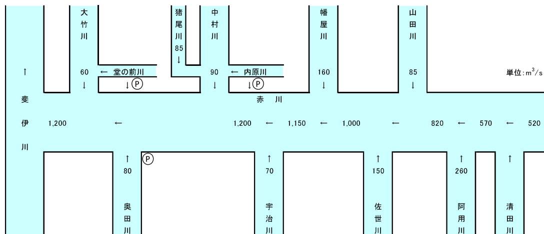
図-4.2 赤川水系流量配分図
