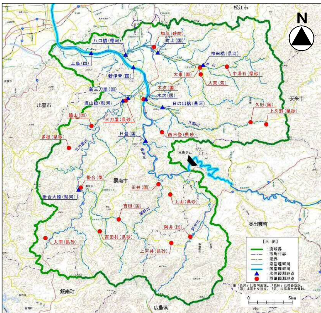
図-3.2 水位及び雨量観測所位置図
