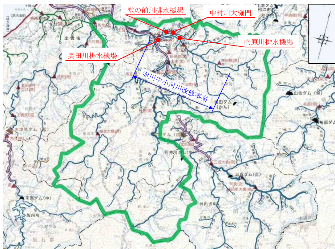
図-4.1 施行位置図
