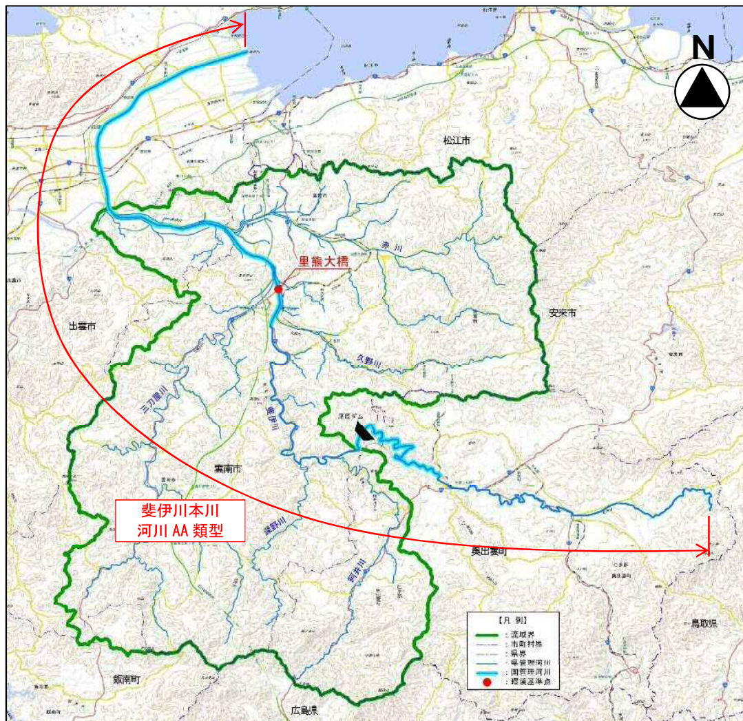
図-3.5 環境基準の類型指定状況と環境基準点
