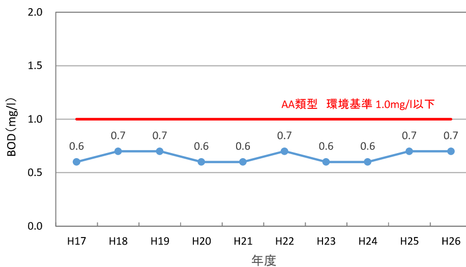
図-3.4 環境基準点・里熊大橋での BOD(75%値)の経年変化
