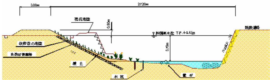
八尾川中流工区 315m 3 /s 区間 (有木川合流点より上流 1km 地点：3k600)
