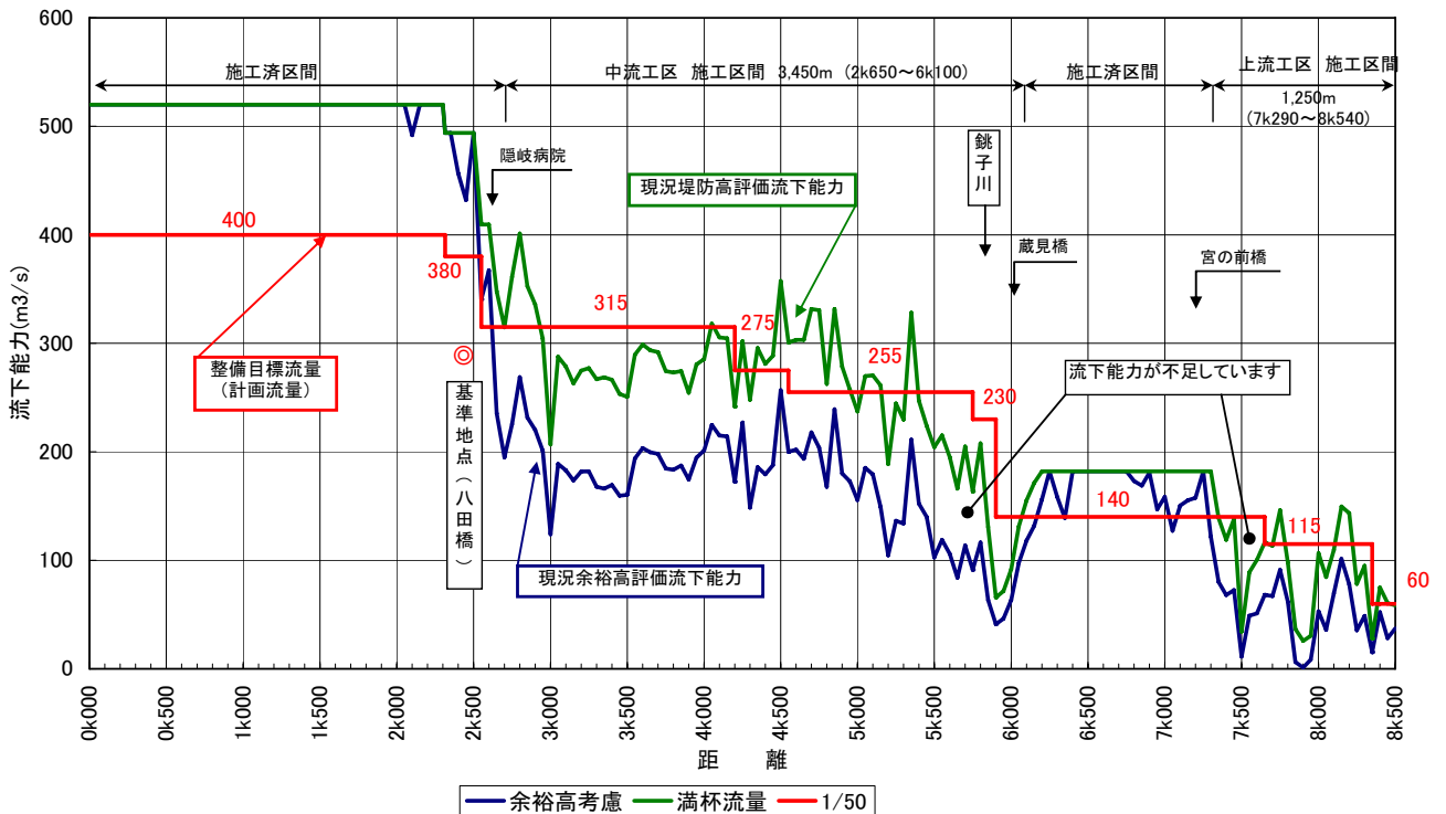
図 3-3 八尾川現況流下能力図
