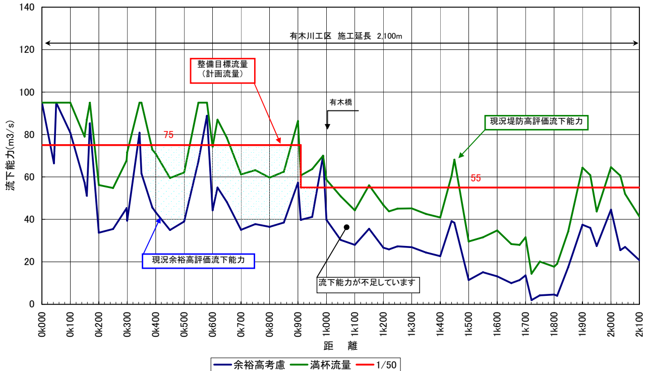
図 3-5 有木川現況流下能力図
