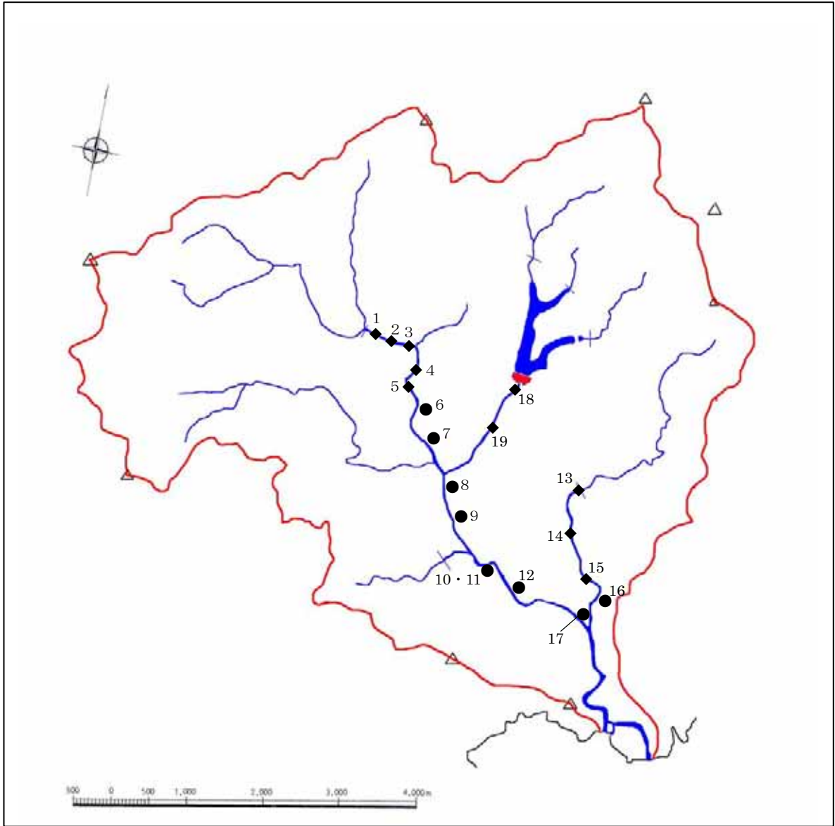
图 1-3 八尾川水系取水位置图
