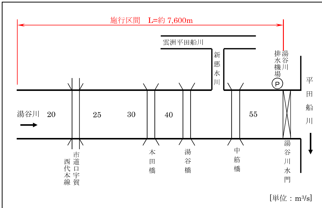
図-4.1.10 整備計画目標流量図
