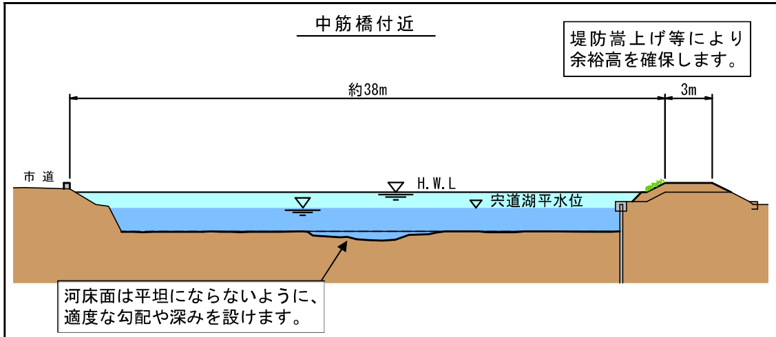
図-4.1.12 標準横断面図 (1)
