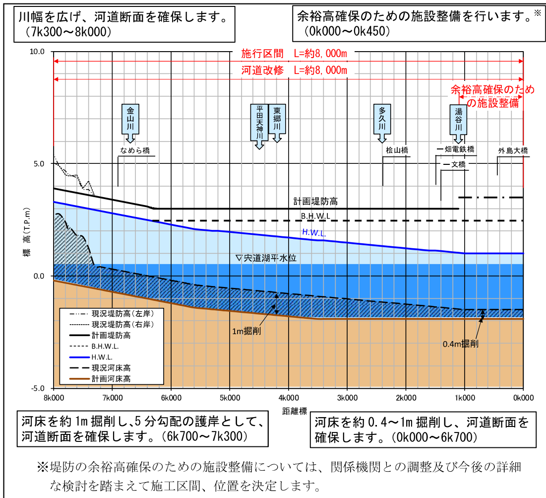
図-4.1.4 縦断面図
