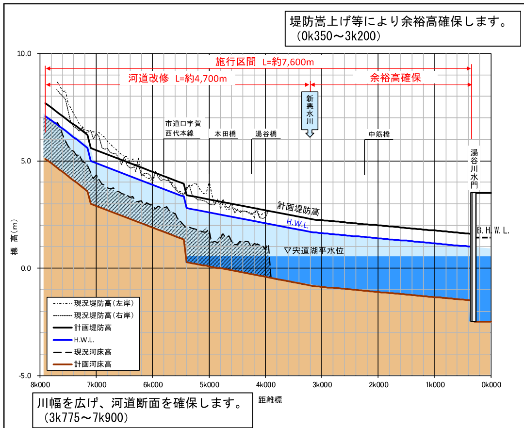
図-4.1.11 縦断面図
