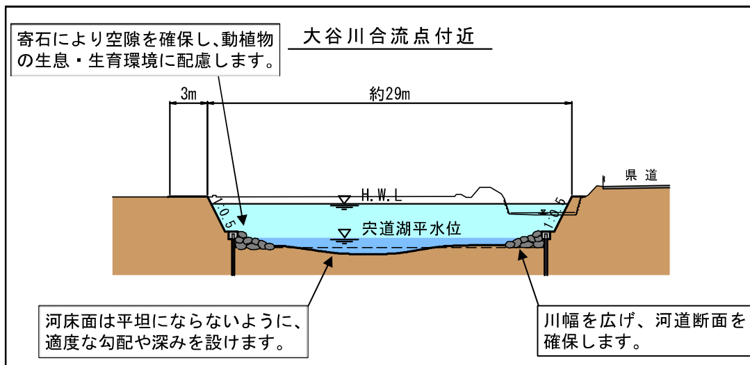
図-4.1.8 標準横断面図 (4)
