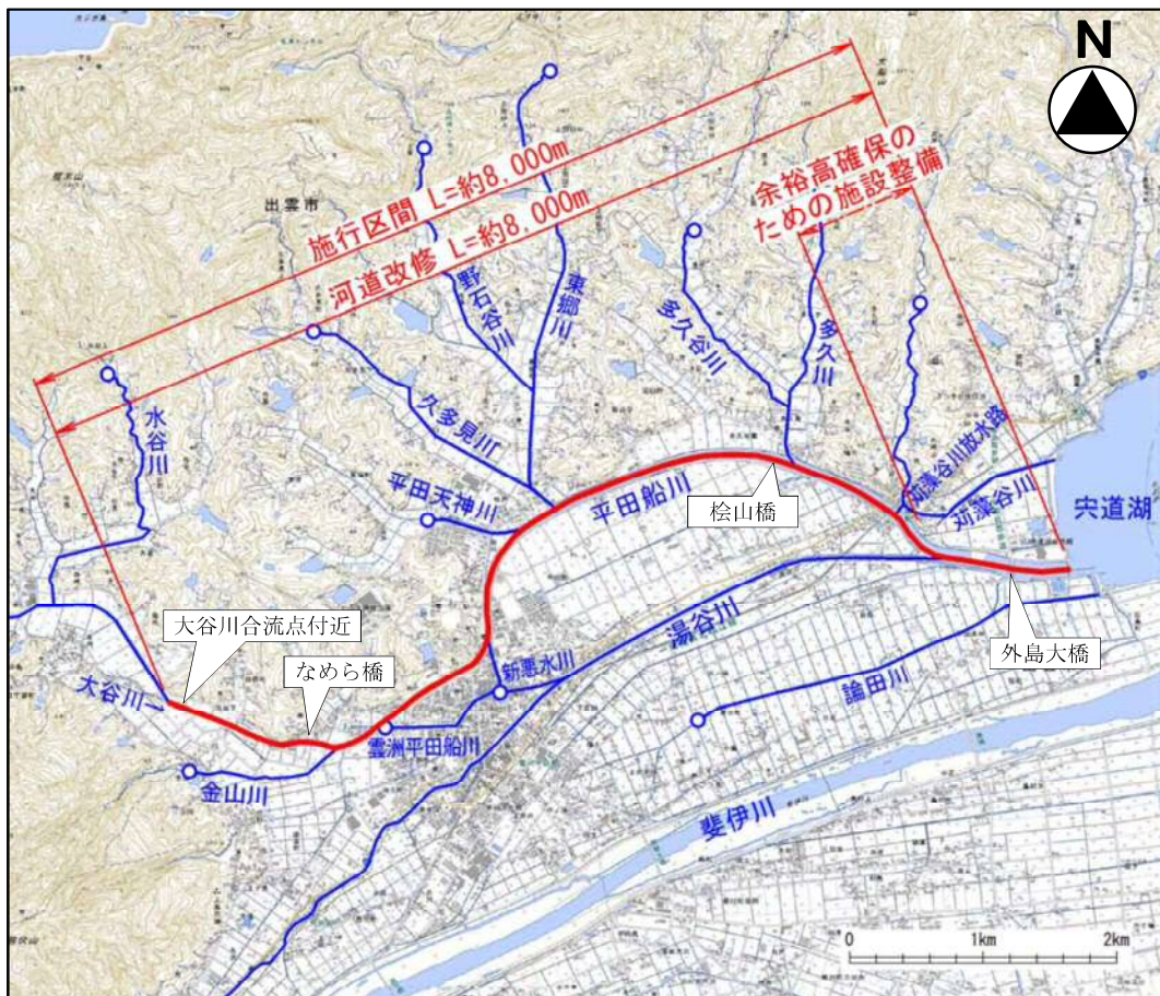
図-4.1.2 平面図
