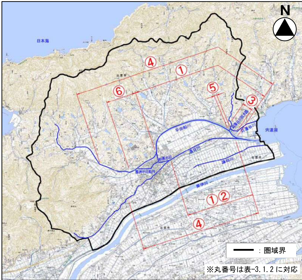
図-3.1.2 主な河川改修事業位置図
