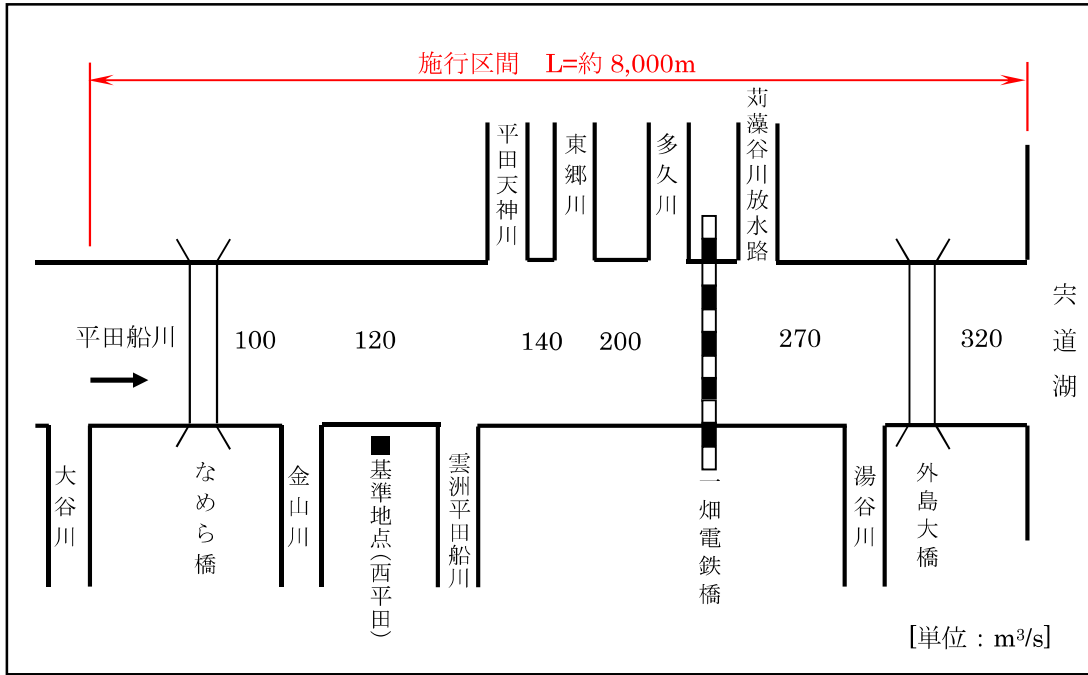
図-4.1.3 整備計画目標流量図
