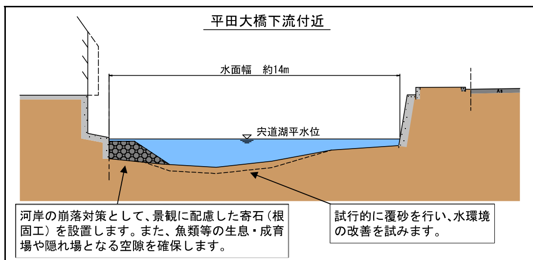
図-4.1.17 横断イメージ図
