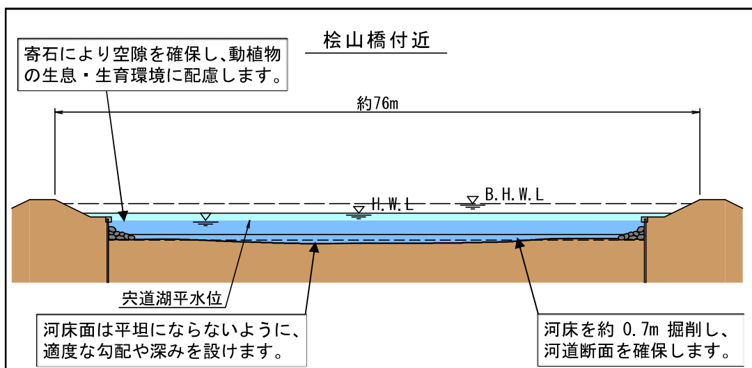
図-4.1.6 標準横断面図 (2)
