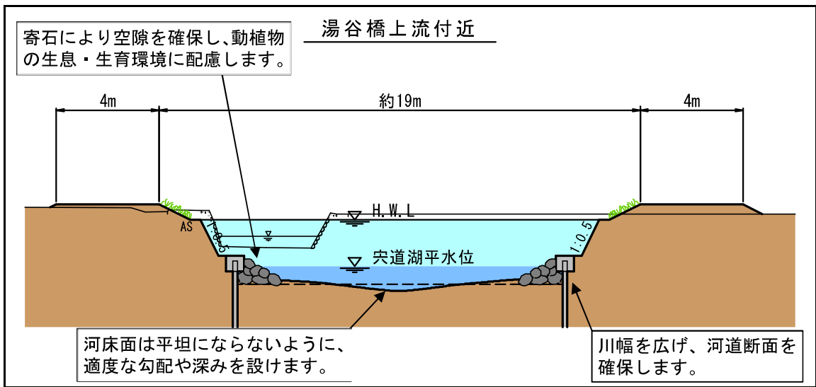
図-4.1.13 標準横断面図 (2)
