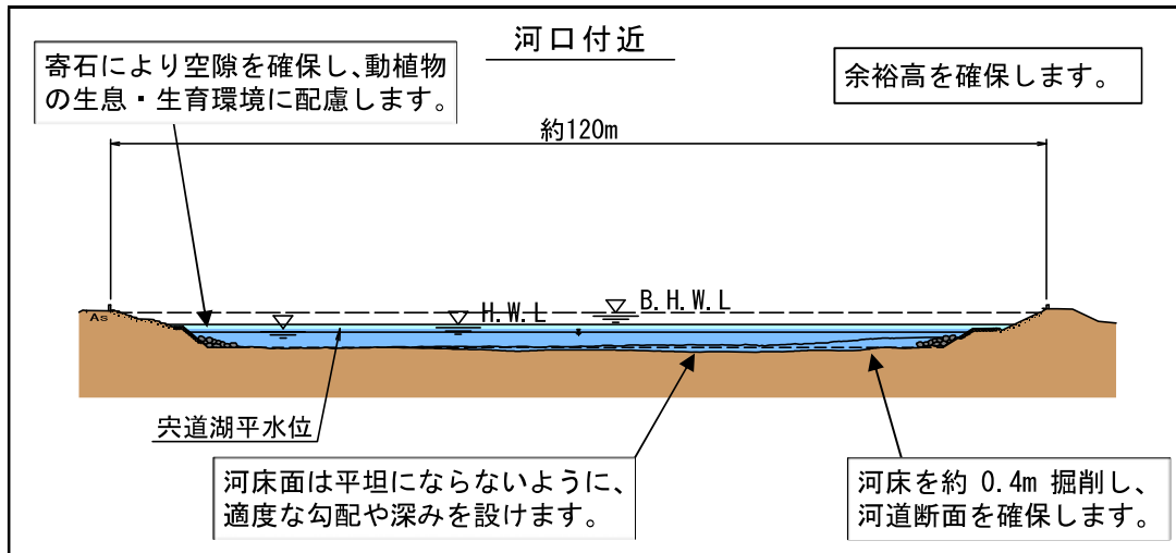
図-4.1.5 標準横断面図 (1)
