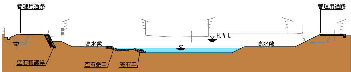
図-3.3.4 糸川屋橋付近代表断面図
