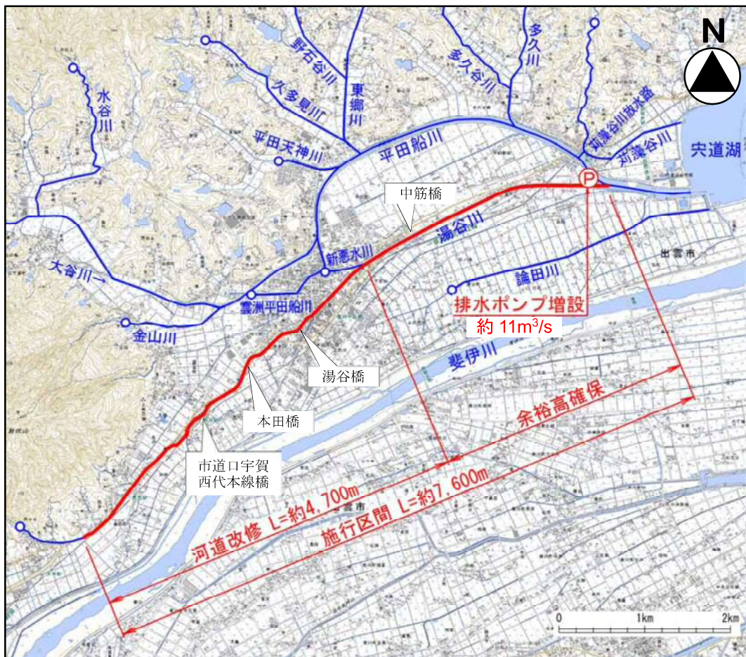
図-4.1.9 平面図
