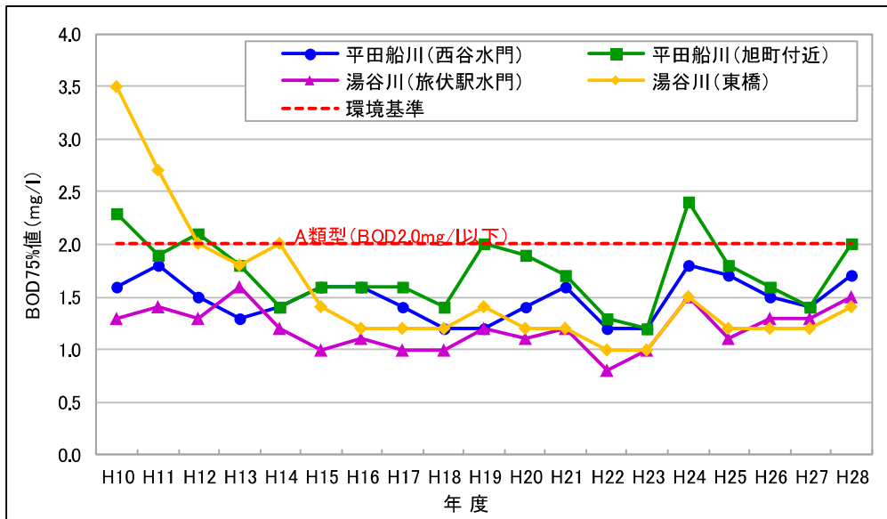
図-3.3.2 BODの推移
