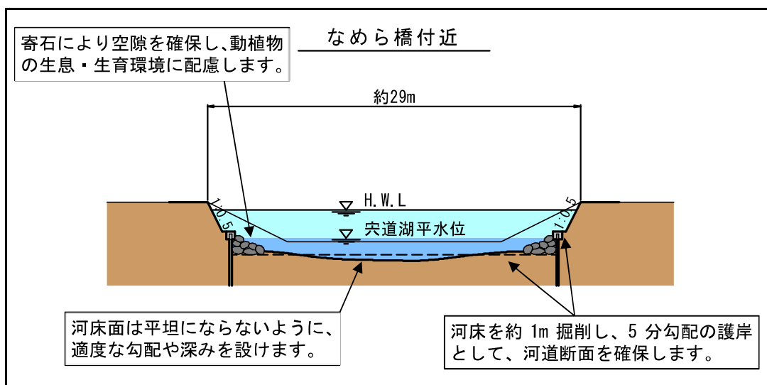
図-4.1.7 標準横断面図 (3)
