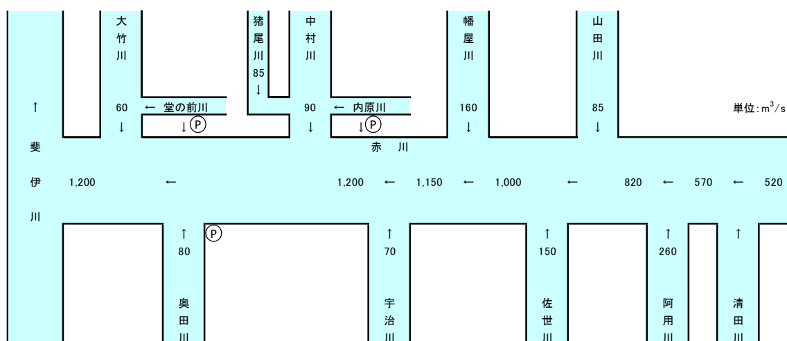
図-4.2 流量配分図 (赤川)
