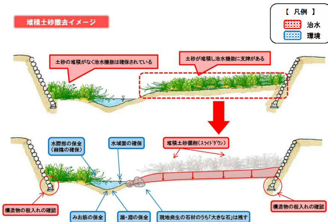
図-4.10 堆積土砂撤去イメージ図
