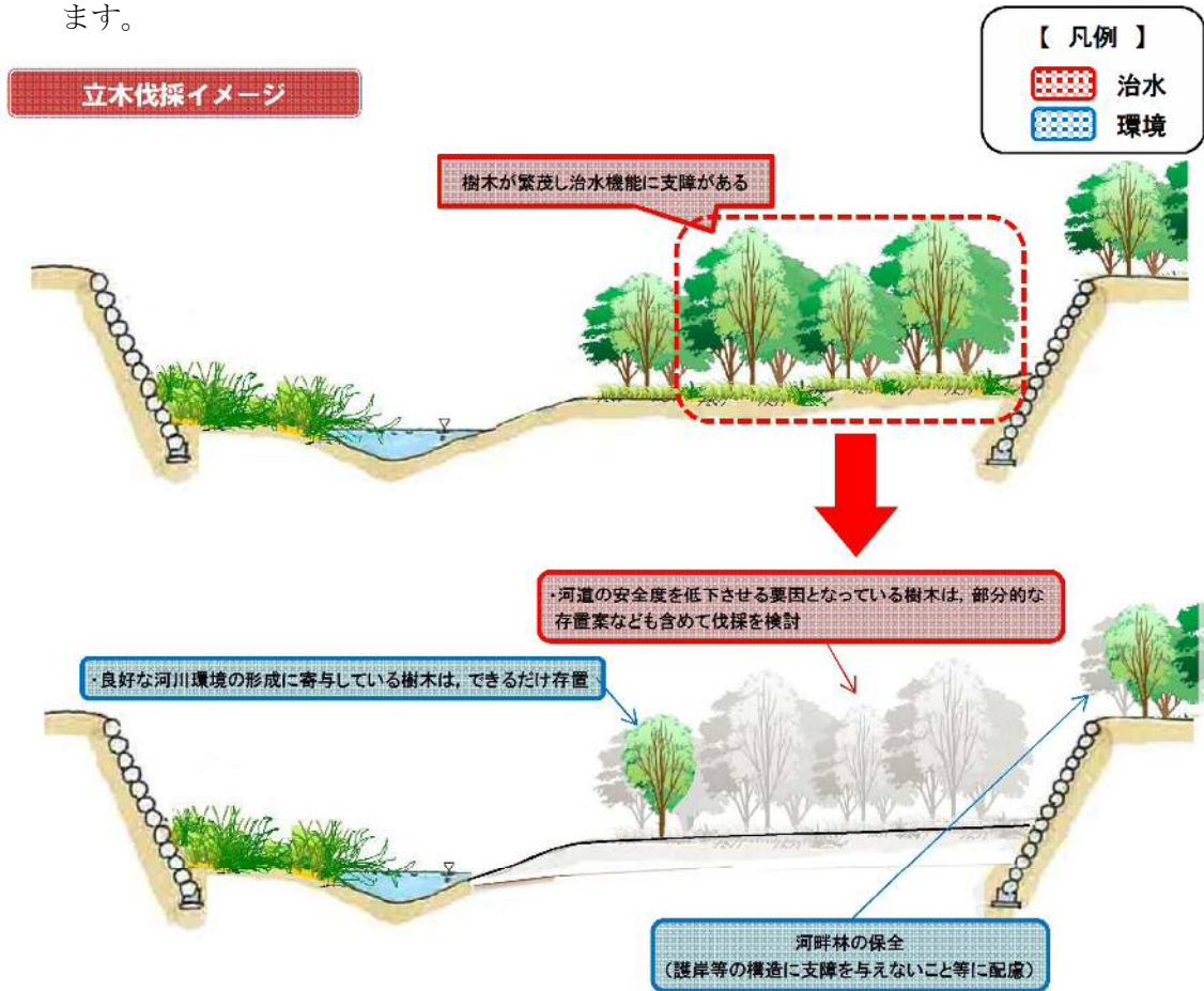
図-4.11 立木伐採イメージ図
