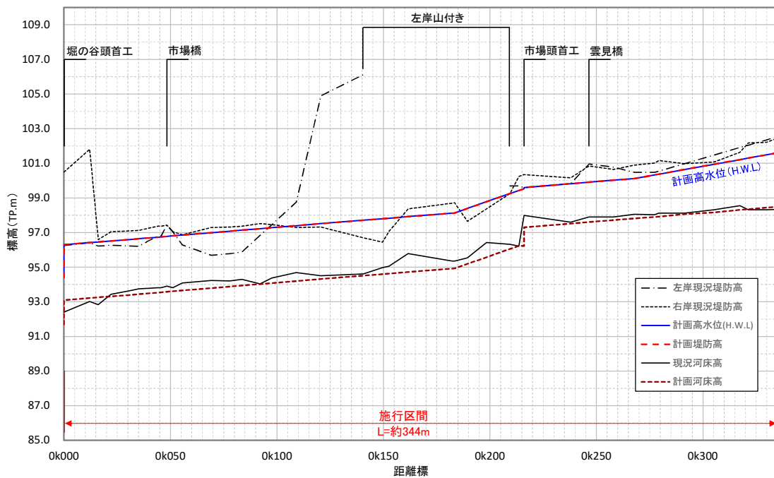
図-4.9 河道の縦断形（飯石川：多久和）
