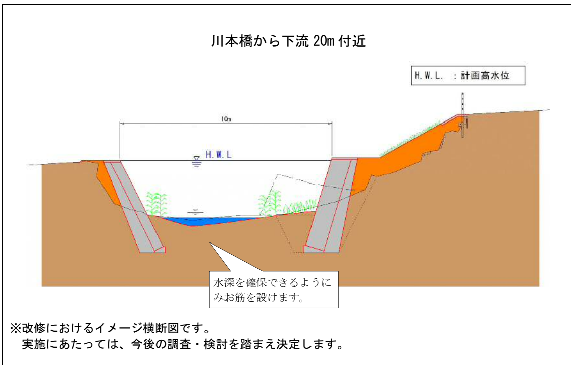
図-4.7 河道の横断形（飯石川：多久和）
