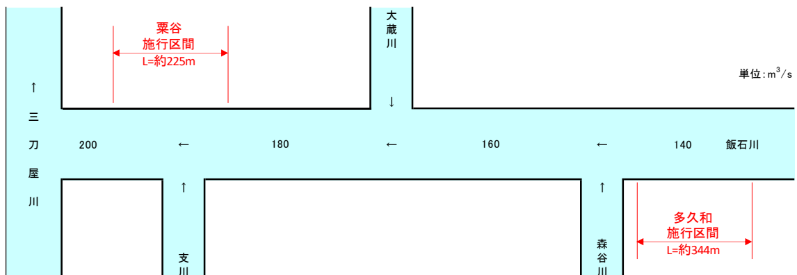
図-4.5 流量配分図（飯石川）
