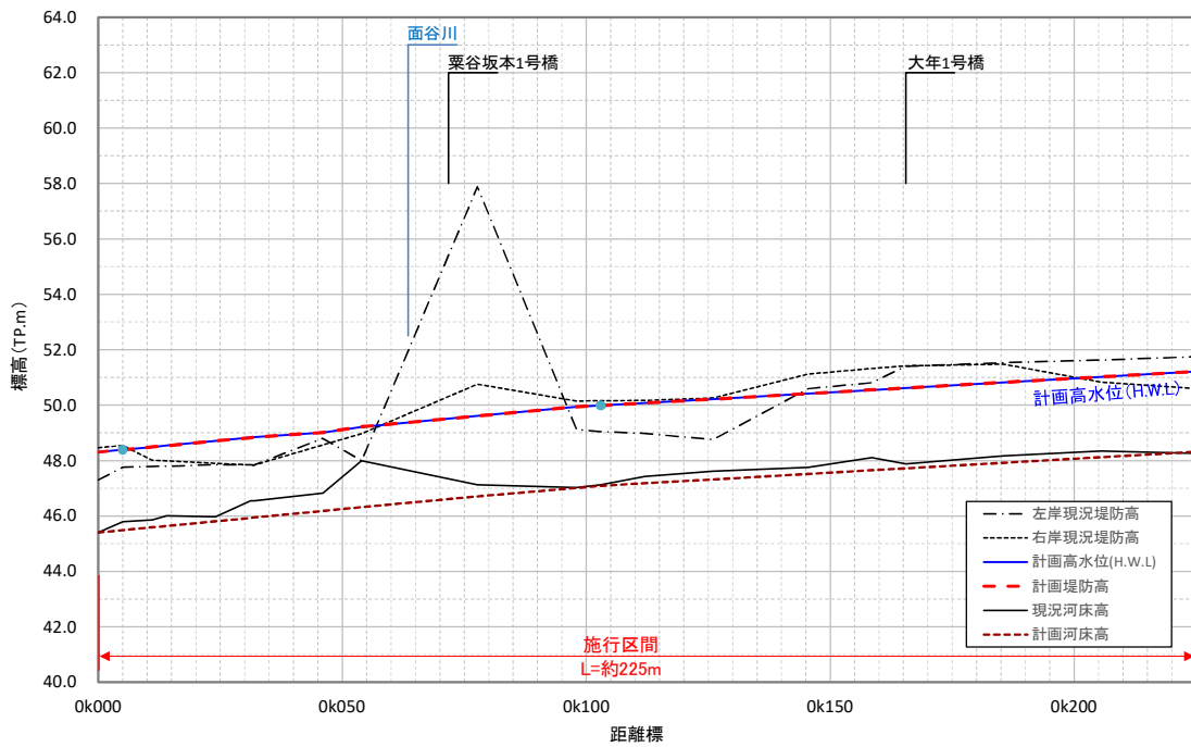
図-4.8 河道の縦断形（飯石川：粟谷）
