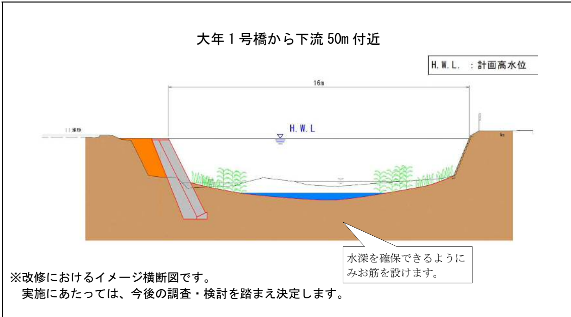
図-4.6 河道の横断形（飯石川：粟谷）
