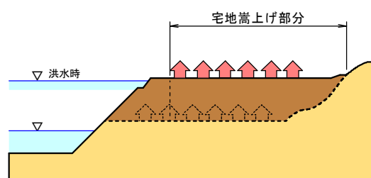
【宅地嵩上げ方式】
