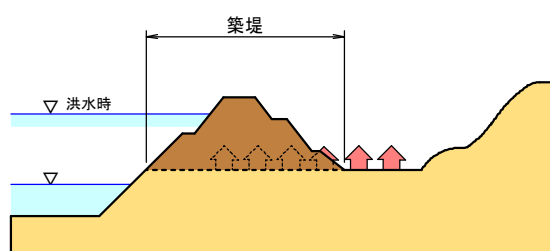
【通常の築堤方式】
