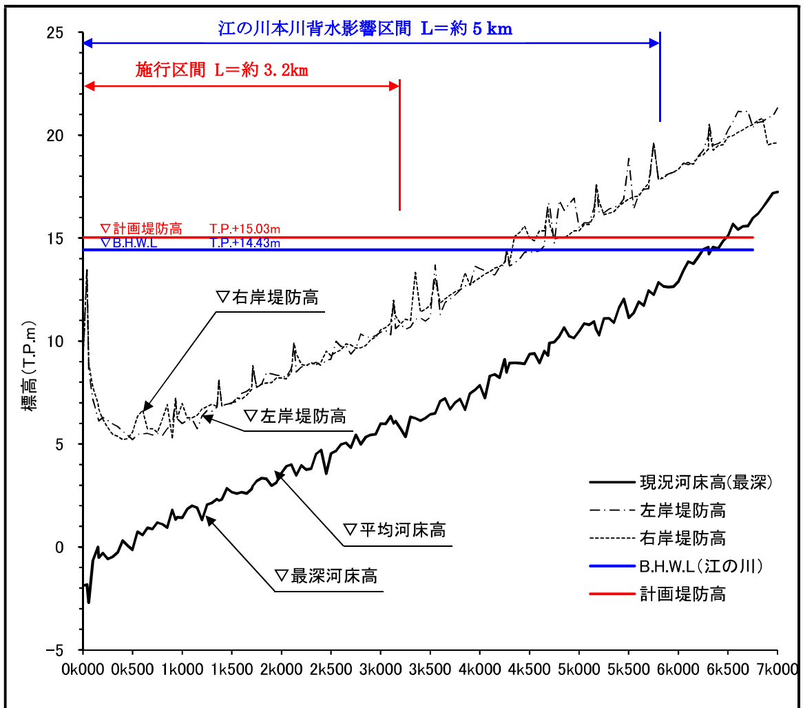
図 4-10 河道の縦断面形 (都治川 (下流部))
