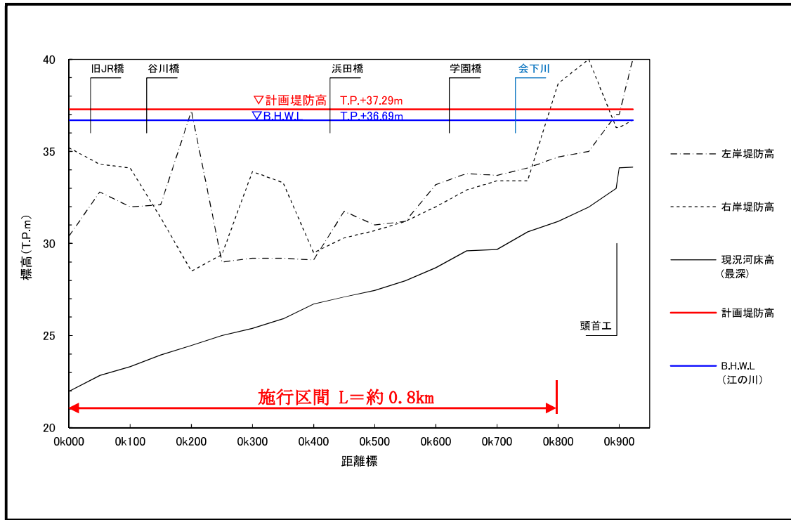
図 4-13 河道の縦断形 (矢谷川)
