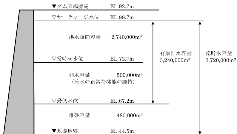
図 4-5 波積ダム貯水池 容量配分図
