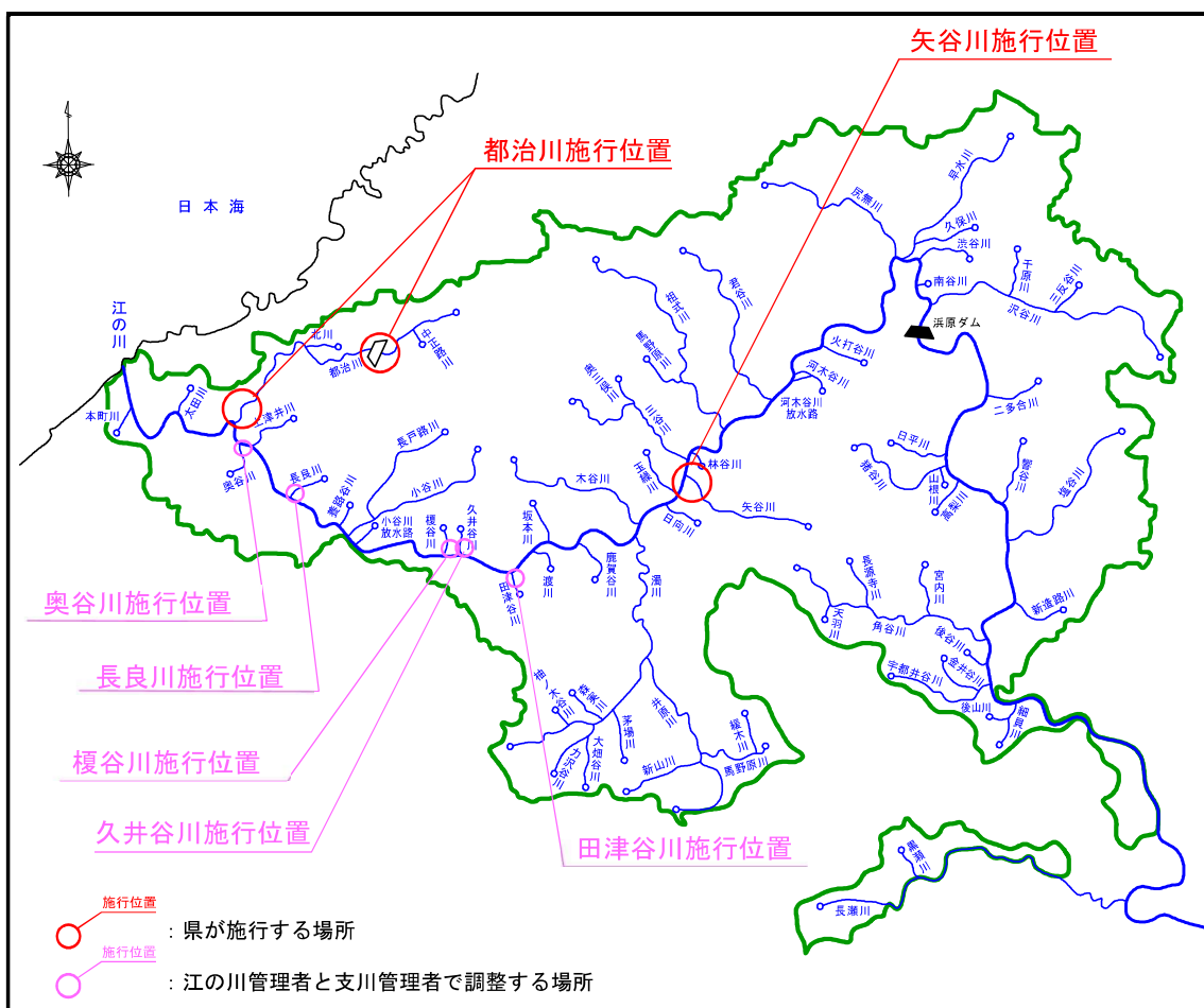
図 4-2 施行区間位置図
