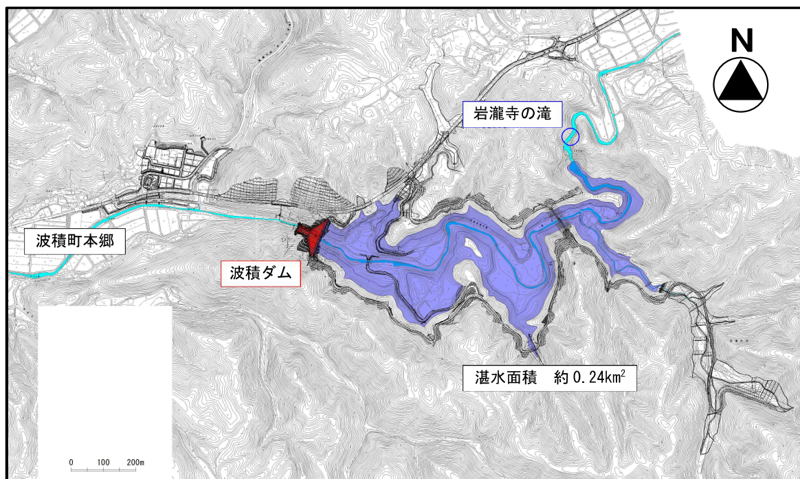
図 4-7 波積ダム 平面図
