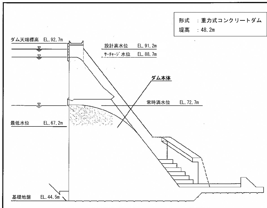
図 4-6 波積ダム建設 標準横断面図
