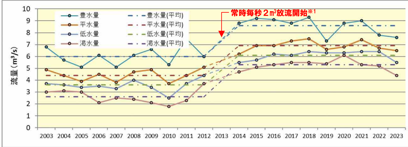
菅田測水所河川流量
