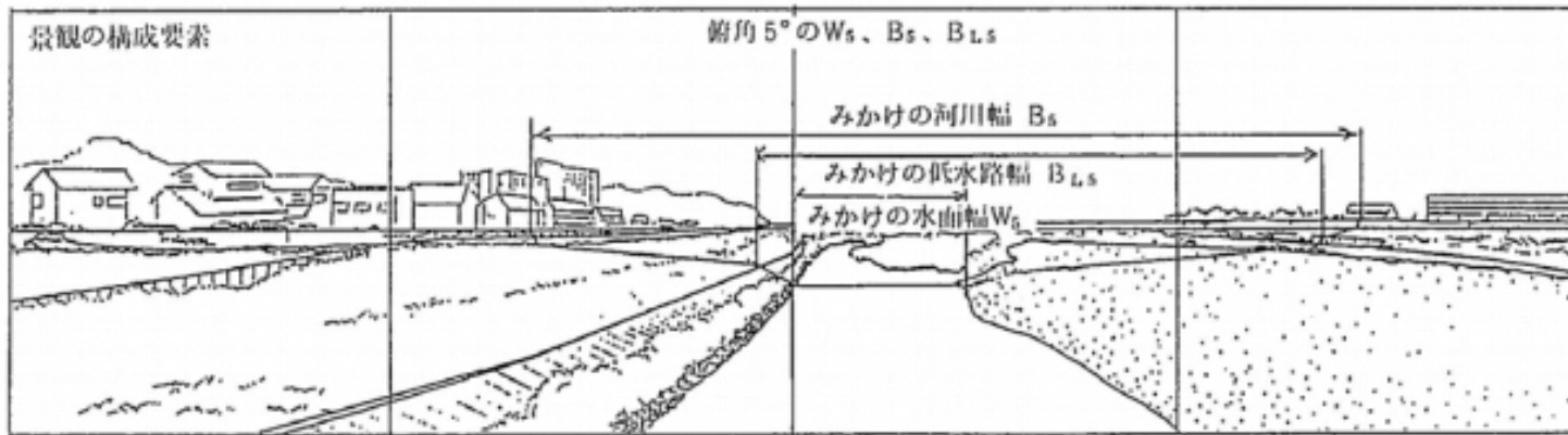
図 パラメータ W/B の算出法
