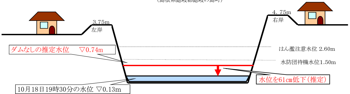
八尾川水位局付近断面図 (島根県隠岐郡隠岐の島町)
