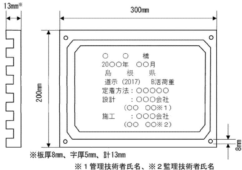
図3-2-2銘板の寸法及び記載事項
