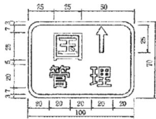
管理紙 (アルミ合金製:100×70) 記号 BS-5-1
