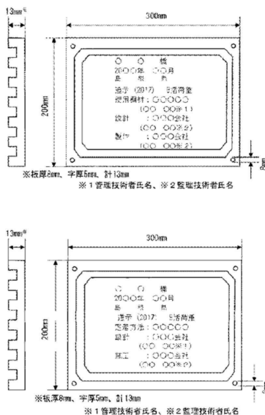
図3-2-2銘板の寸法及び記載事項
