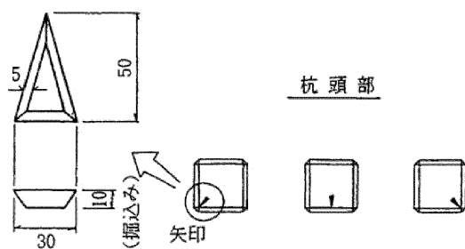
矢印詳細図（掘込式）
