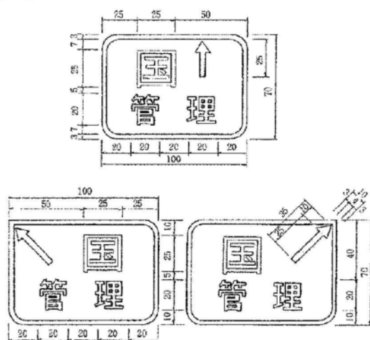
管理紙（アルミ合金製：100×70） 記号 BS-5-1
