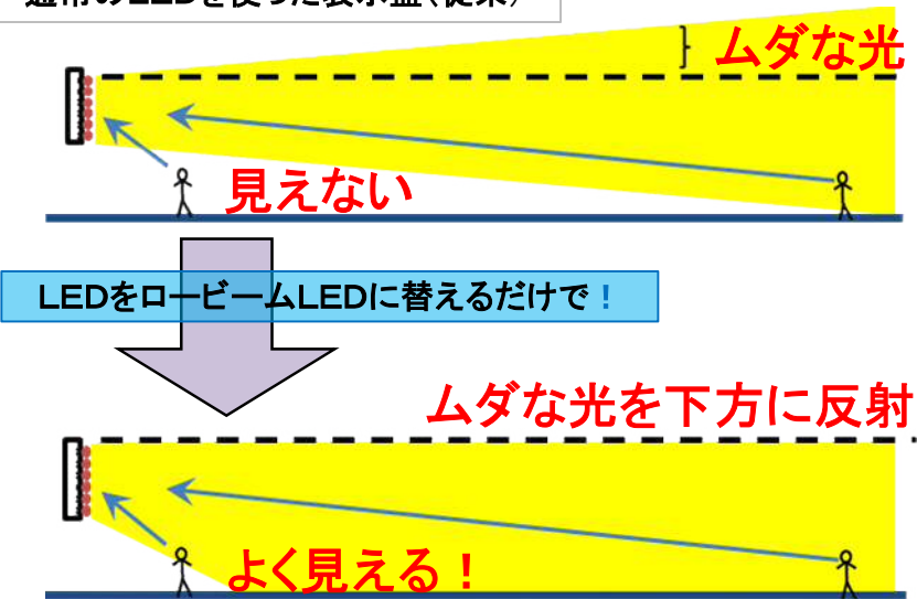
通常のLEDを使った表示盤(従来)
