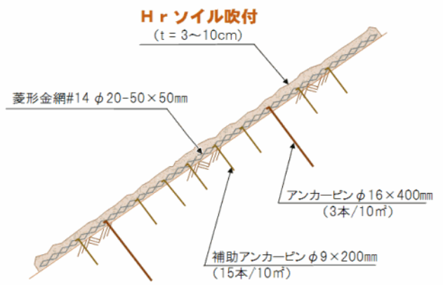
道路工事 切土法面の防草工 【本設タイプ】
