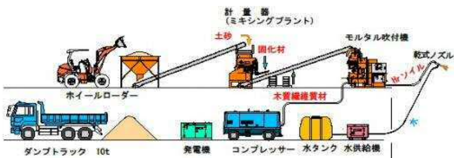
【乾式吹付設備】
