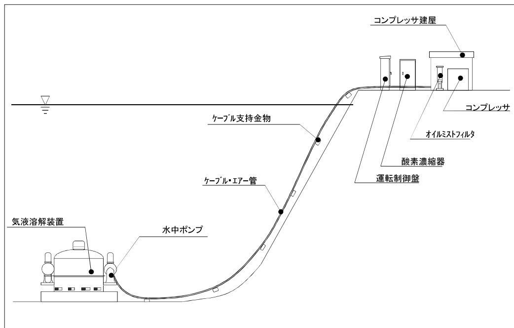
設置イメージ 浅瀬方式
