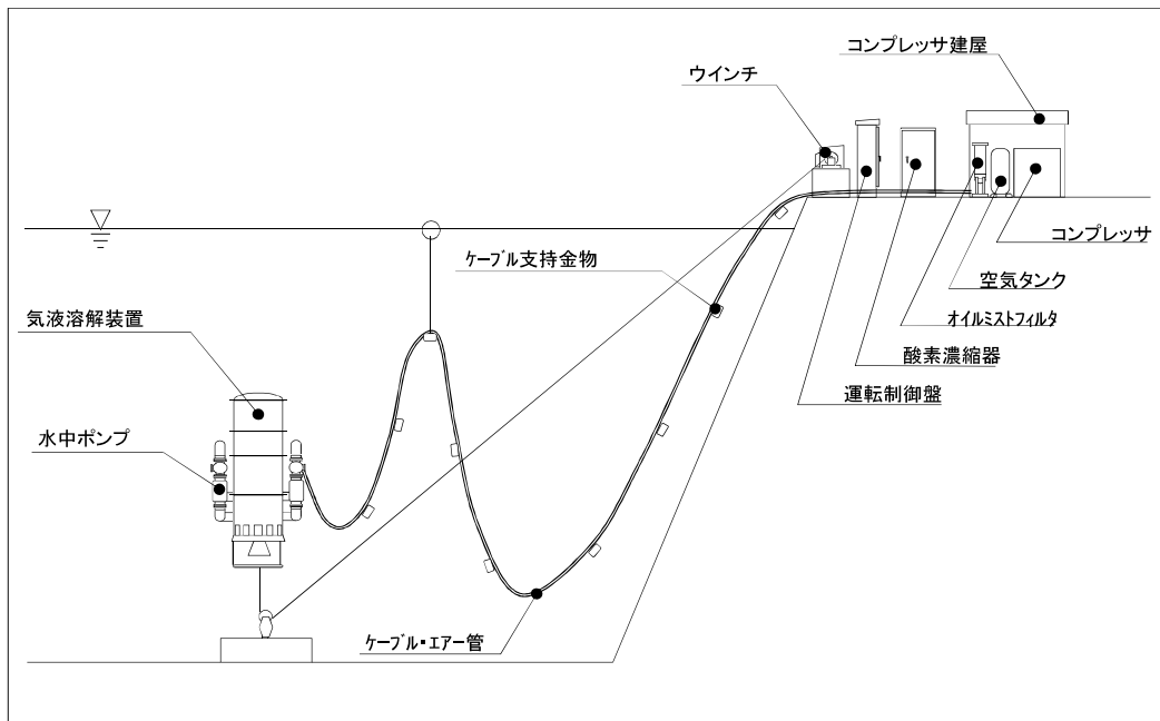
設置イメージ アンカー方式
