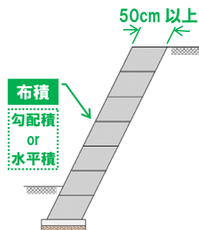
タイプ3: もたれ式擁壁に準じた構造の大型ブロック積擁壁
