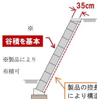
タイプ1-②: 積みブロックの控長を 35cm のまま大型化したブロック積擁壁
