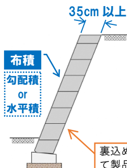
タイプ2: 通常のブロック積(石積)擁壁に準じた構造の大型ブロック積擁壁
