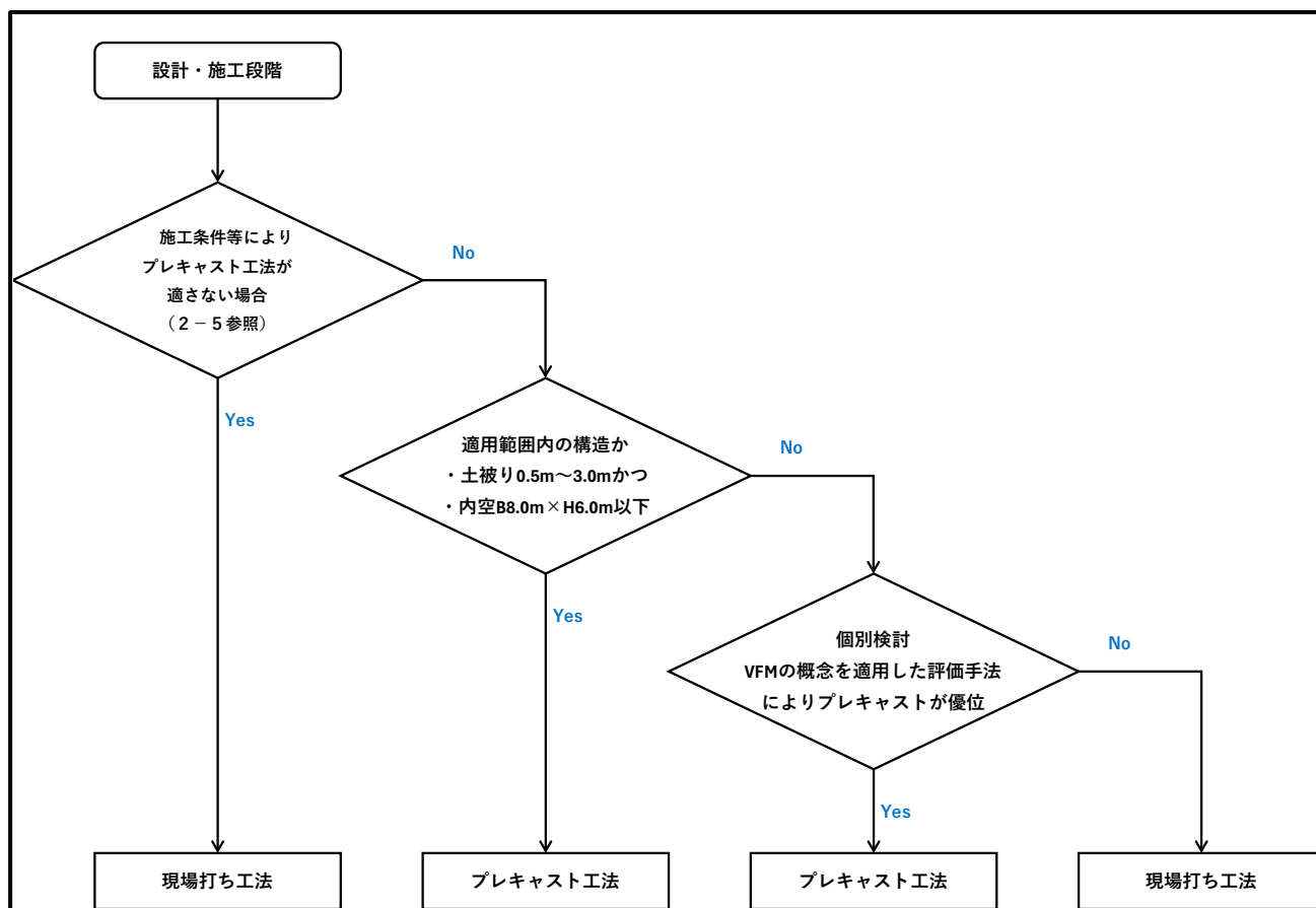
図 2-1. 工法選定フロー
