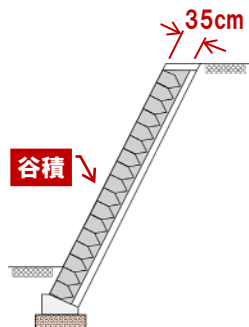
タイプ1-①: 通常のブロック積(石積)擁壁
