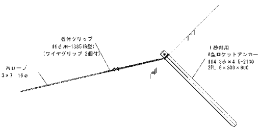
(土砂部の場合)
