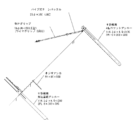
(土砂部の場合)
