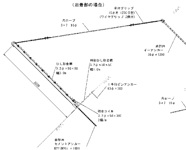
(岩着部の場合)
