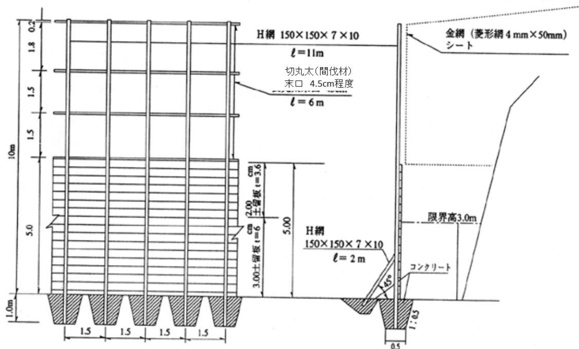
※安全の為ステー（アンカー）を取るのが良い。
