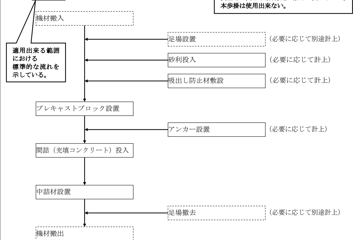
図1-1 施工フロー
