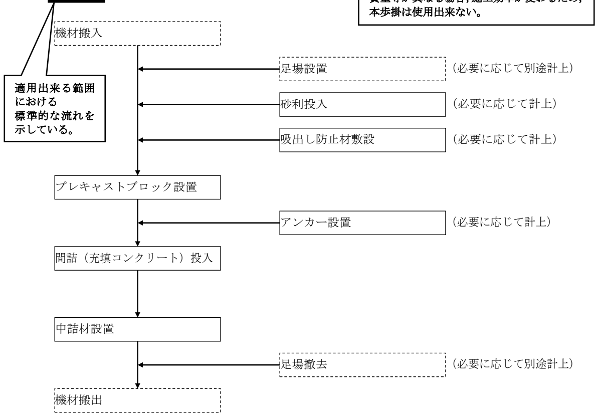
図1-1 施工フロー
