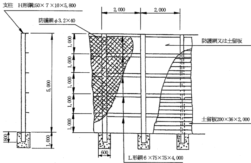
側面図
