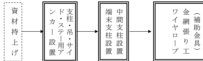
図2-1 施工フロー
