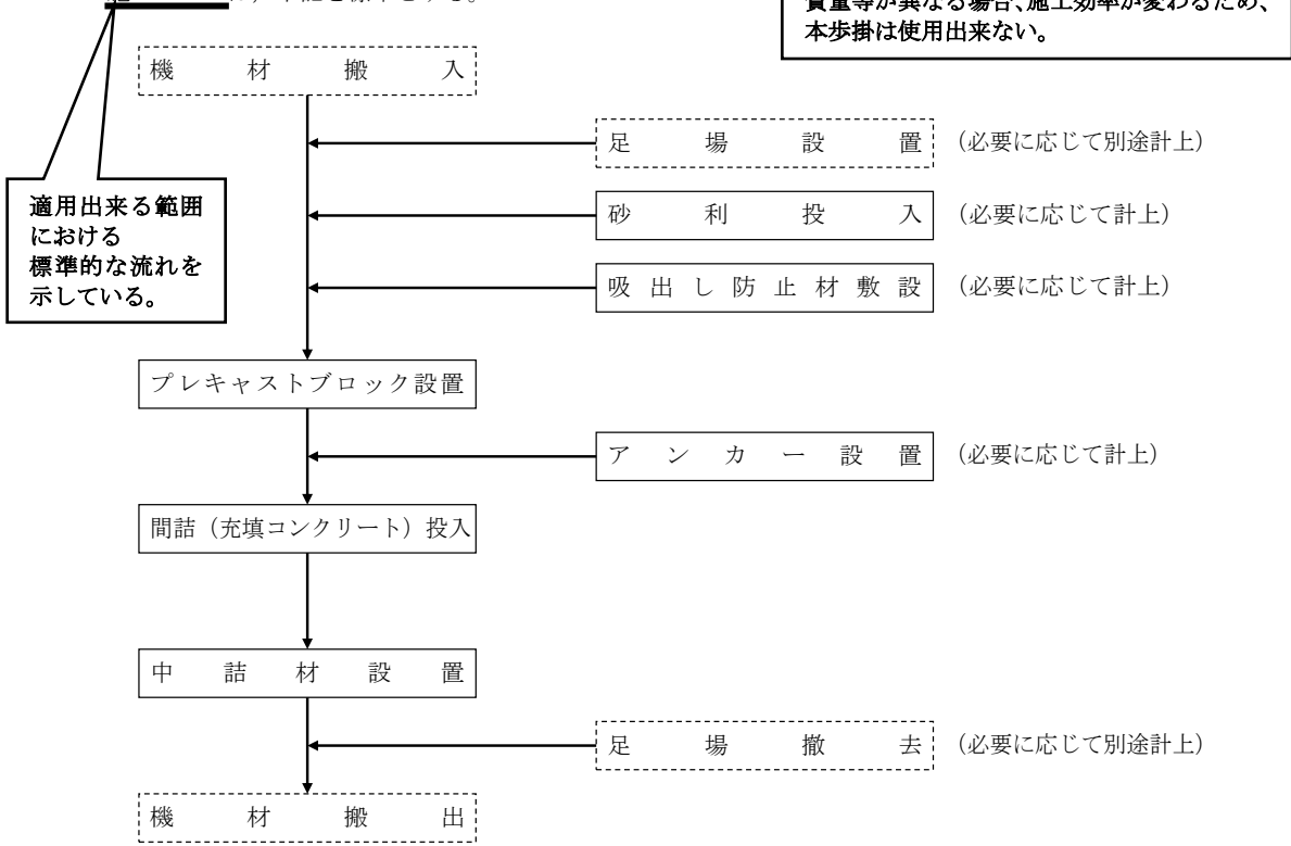
図1.1 施工フロー
