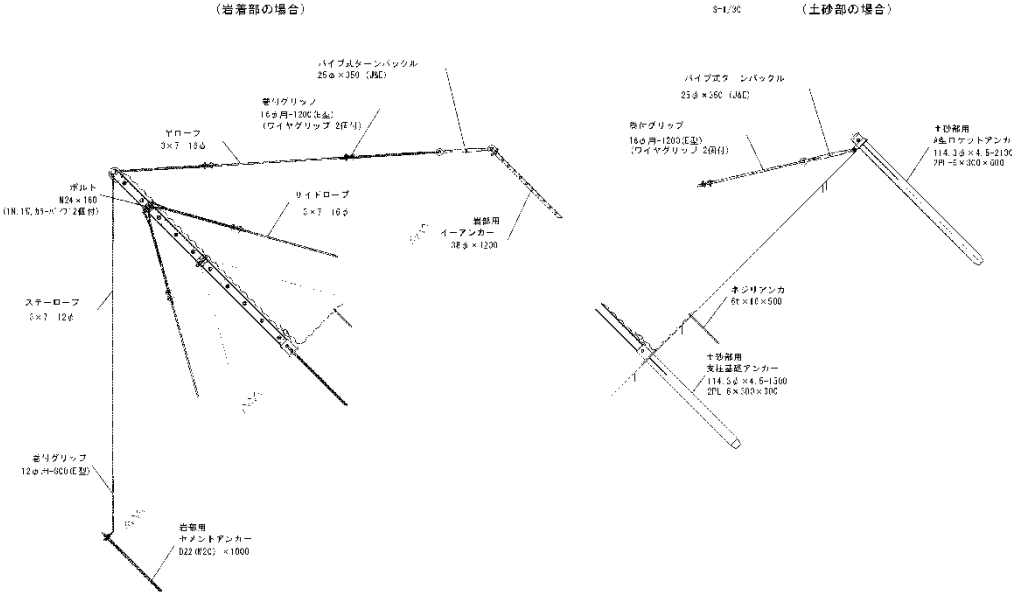
端末支柱断面図
