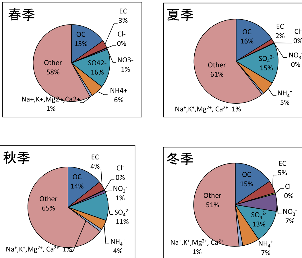
図4. 平成30年度 PM2.5季節別平均成分割合
