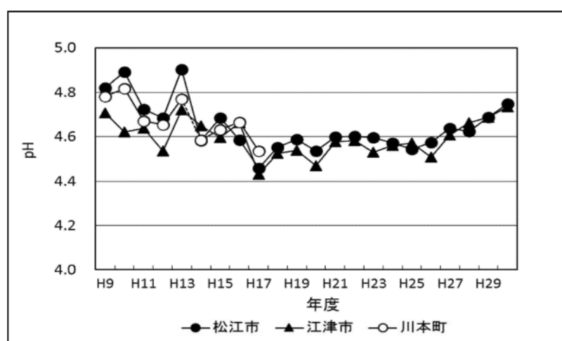
図1 pH年平均値の経年変化
