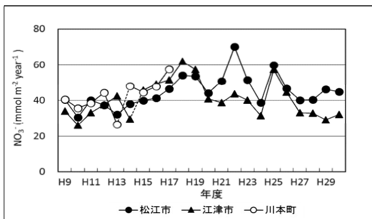
図3 NO 3 - 年間沈着量の経年変化
