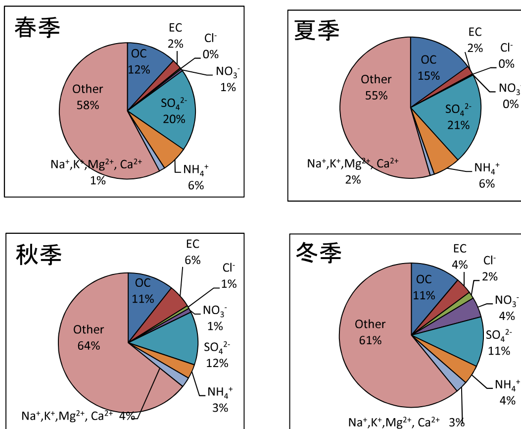
図2. 平成30年度 PM2.5季節別平均成分割合
