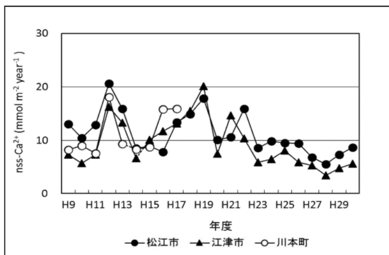
図5 nss-Ca 2+ 年間沈着量の経年変化
