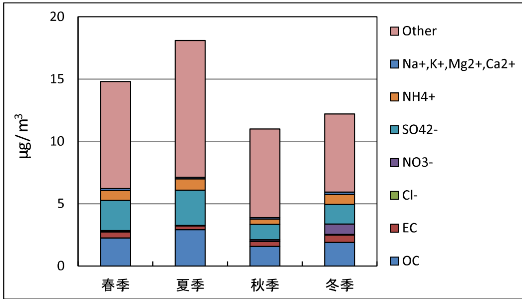
図3. 平成30年度 PM2.5季節別平均成分濃度
