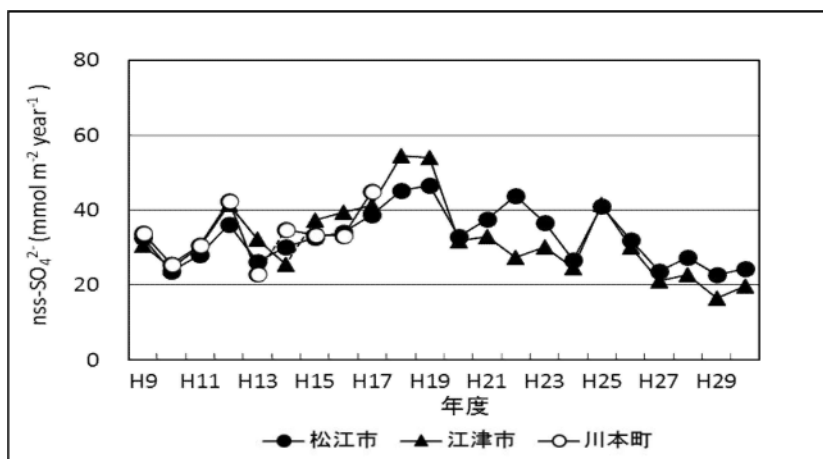
図2 nss-SO 4 2- 年間沈着量の経年変化
