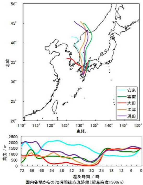
図5 2018年4月29日16時の後方流跡線解析結果
