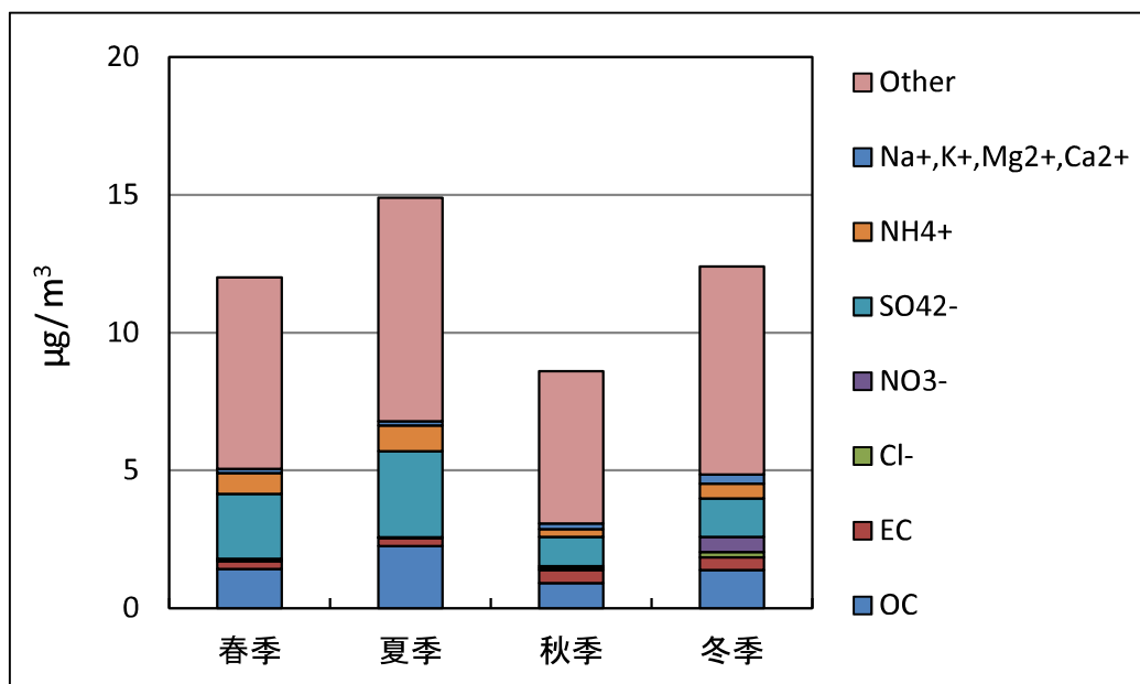
図1. 平成30年度 PM2.5季節別平均成分濃度
