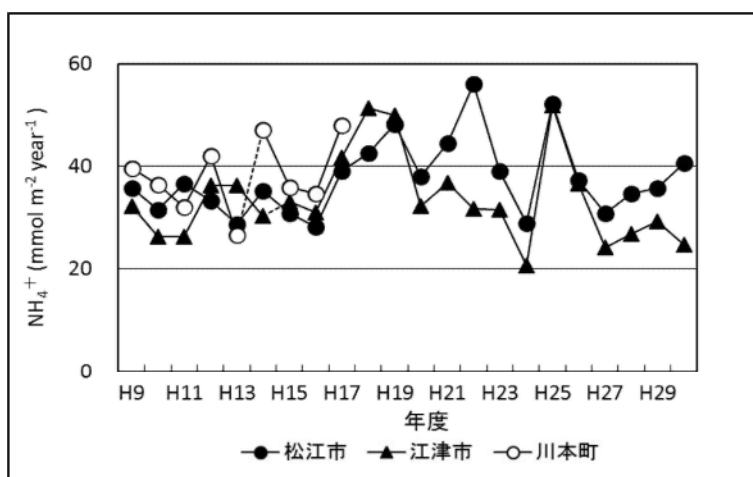
図4 NH 4 + 年間沈着量の経年変化
