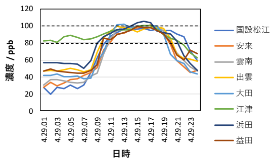
図3 2018年4月29日のOx濃度の経時変化
