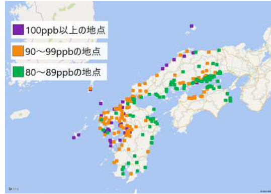
図4 2018年4月29日に中国・四国・九州地方で80ppb以上の高濃度Oxが観測された地点
