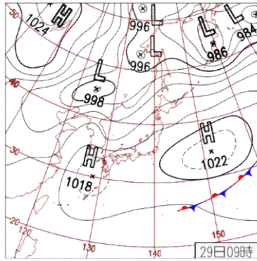
図1 2018年4月29日9時の気圧配置図 (気象庁ホームページ日々の天気図より転載)
