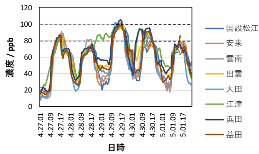
図2 2018年4月27日～5月1日のOx濃度の経時変化
