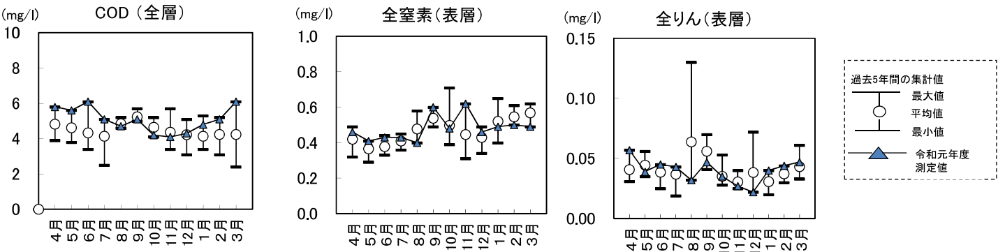
図. 矢道湖湖心における令和元年度水質測定値の経月変化
