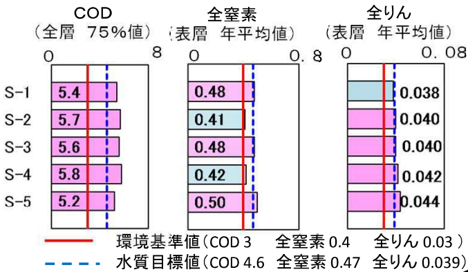
図1-2. 矢道湖の環境基準点の測定結果
