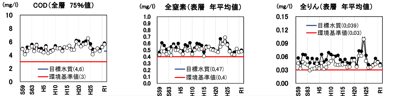
図1-3. 矢道湖の水質の経年変化
