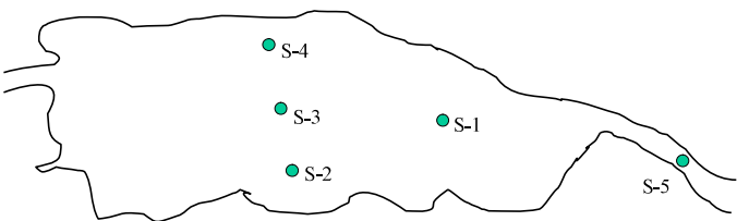
図1-1. 矢道湖の測定地点図
