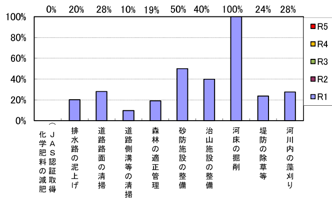
図3-2. 各種施策の進捗状況 (注1)
