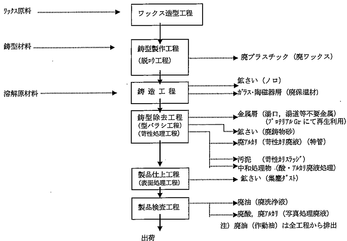
図1 精密鋳造品製造フローシート
