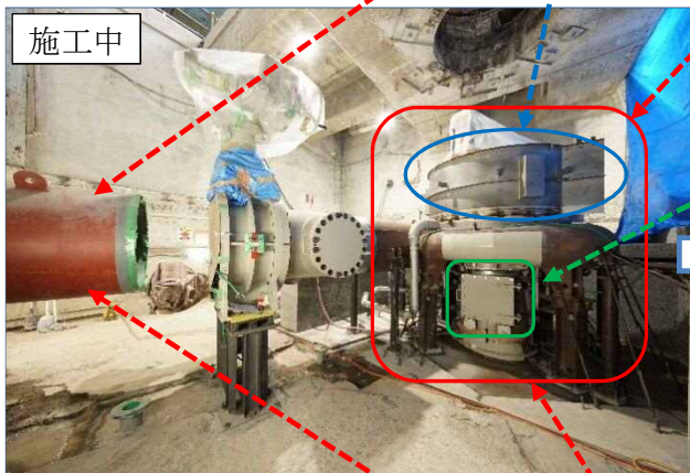
水圧鉄管・水車外部・入口弁 (地下3階)
