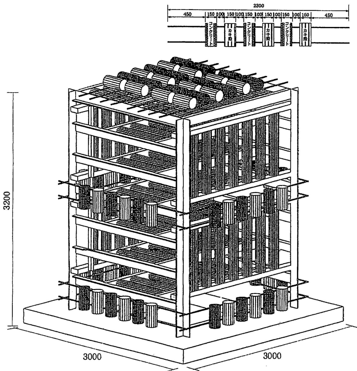
テストピース組立図
