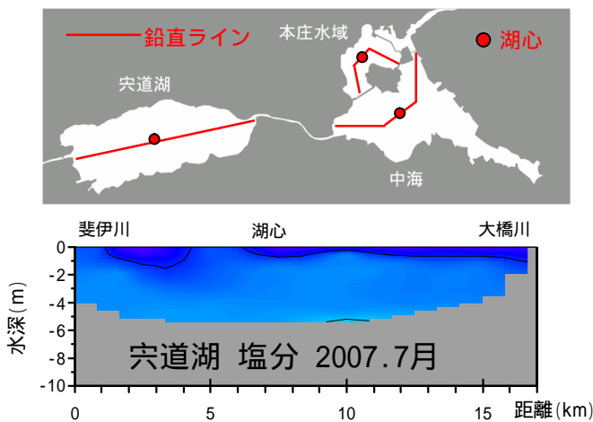
塩分 鉛直分布
