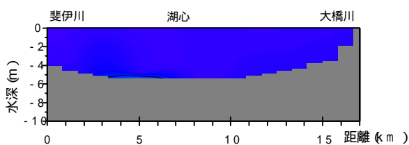
宍道湖 塩分 2004.1月
